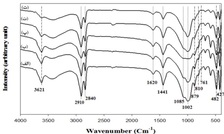
شکل ۳ طیف‌های FTIR خاک رس الف): پیش از آسیاکاری، و پس از آسیاکاری به مدت ب) ۱ ساعت، پ) ۲٫۵ ساعت، ت) ۱۰ ساعت و ث) ۴۰ ساعت.
