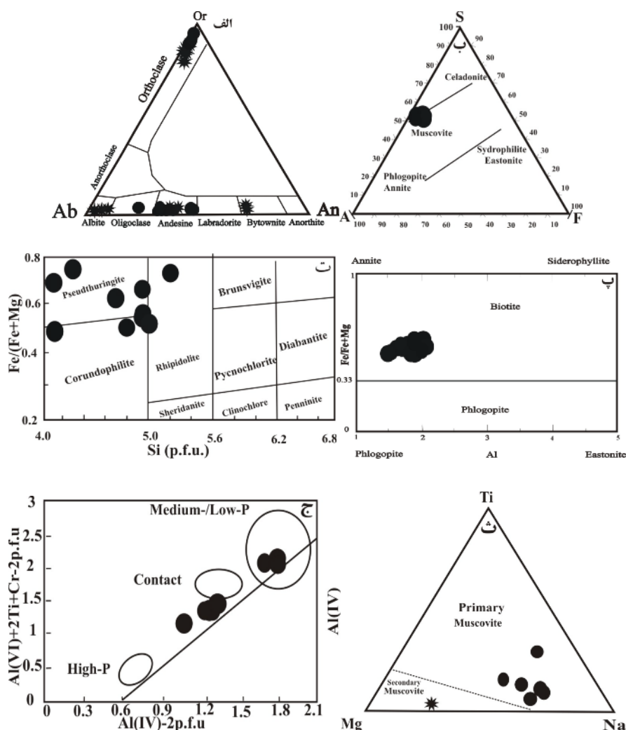
شکل ۶ الف) ترکیب فلدسپارها در زینولیت‌های منطقه‌ی آستانه روی نمودار Ab-Or-An [۱۴] ب) ترکیب شیمیایی مسکوویت روی نمودار سه تایی (\text{SAF})\text{SiO}_2\text{-FeO-Al}_2\text{O}_3 [۱۵] پ) رده‌بندی شیمیایی میکاها در سنگ‌های مورد بررسی [۱۴، ۱۰] ت) نمودار \text{Fe}^{+2}/\text{Fe}^{+2}+\text{Mg} نسبت به Si در کلریت‌ها [۱۱] ث) موقعیت ترکیب موسکوویت‌های مورد مطالعه [۱۶] ج) ترکیب شیمیایی کلریت‌ها روی نمودار \text{Al}^{(\text{VI})}+2\text{Ti}+\text{Cr}-2 در برابر \text{Al}^{(\text{IV})}-2 ، خط ربط نشان‌دهنده جانشینی چرماک در منطقه‌های مختلف دگرگونی است [۱۲].
