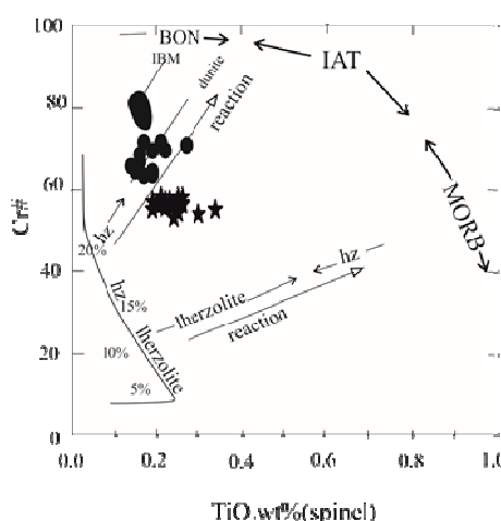
شکل ۷ تغییرات Cr# در مقابل \text{TiO}_2 اسپینل‌های دونیت‌های پیوسته و دایک‌های دونیتی در دو گستره‌ی مجزا قرار می‌گیرند. (FMM = گوشته مورب بارور، IBM = ایزوبونین ماریانا، IAT = تولئیت‌های جزایر قوسی، IBM = بونینیت) [۱۴، ۱۵].
