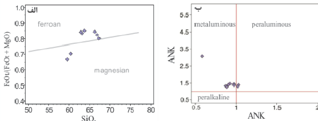
شکل ۳ الف) نمودار ANK (Molar K_2O + Na_2O / Al_2O_3 ) در برابر ACNK (Molar Al_2O_3 / CaO + K_2O + Na_2O ). ب) FeOt / (FeOt + MgO) در برابر SiO_2 (wt%) [۱۵].
