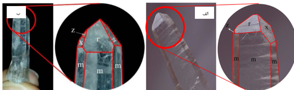
شکل ۴ (الف) موقعیت سطوح r و z در کوارتز معمولی، (ب) تعیین راست‌گرد و چپ‌گرد بودن کوارتز با استفاده از سطوح s, x [۸].
