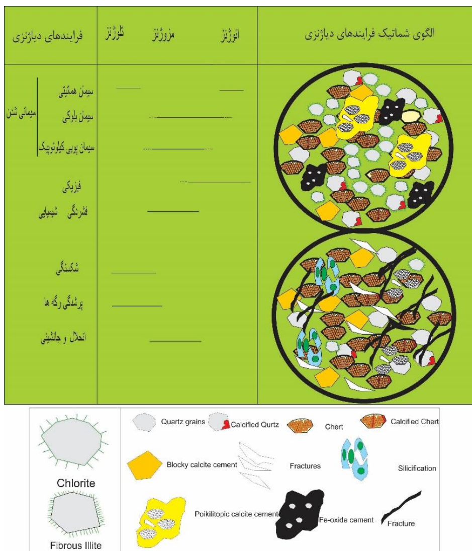
شکل ۹ توالی پارائنتیکی سنگ‌های سیلیسی‌آواری سازند امیران به همراه طرحواره نشان‌دهنده اثر کانی‌های رسی خودزا با شکل پوشاننده ذره‌ها در منطقه مورد بررسی.
