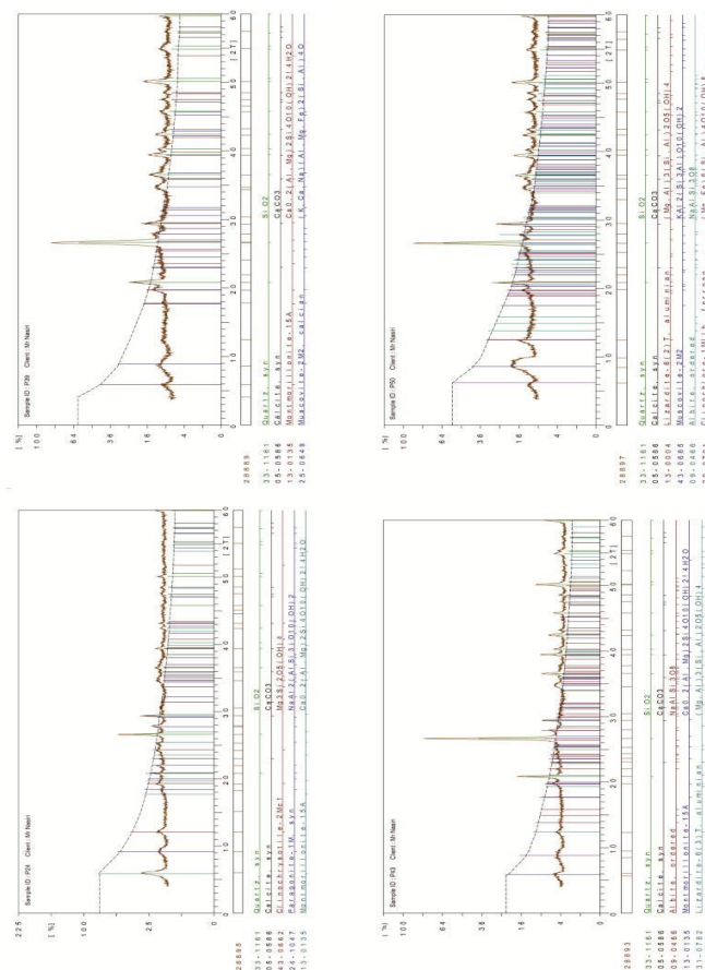
شکل ۵ نتایج XRD برای شیل‌های سازند امیران در برش پیرشمس‌الدین.
