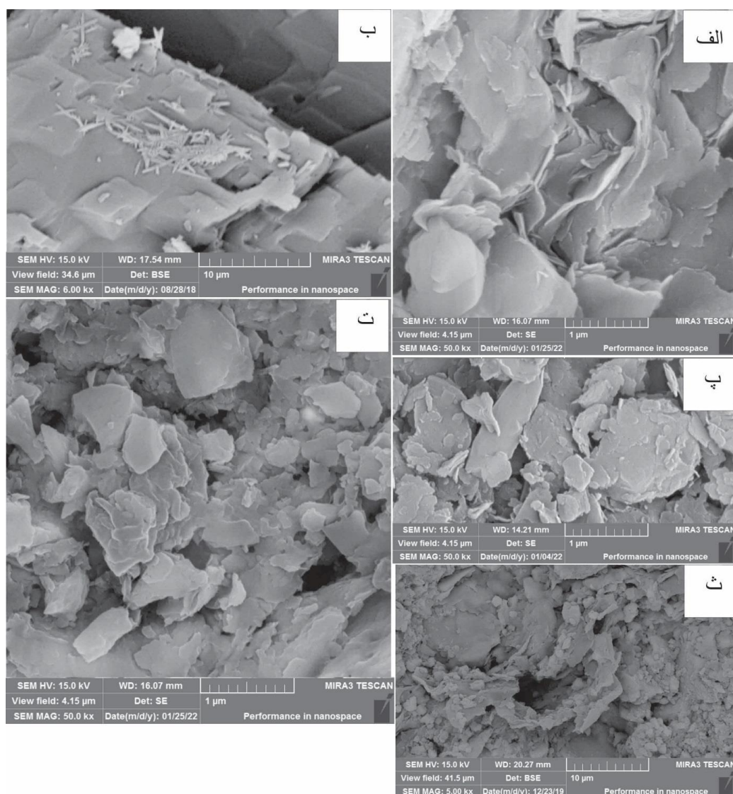
شکل ۸ تصاویر میکروسکوپ الکترونی روبشی (SEM) کانی‌های رسی: الف- پالی‌گورسکیت الیافی و کشیده. ب) کانی رسی ایلیت به شکل سوزنی که از دگرسانی فلسپات بوجود می‌آید، پ و ت) کانی اسمکتیت به شکل ذره‌های پف‌کرده، گل مانند، تودرتو و کرکی شکل که اغلب برای گروه اسمکتیت است، ث) کانی رسی مونت‌موریلونیت.
