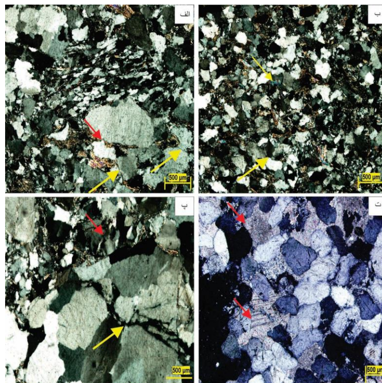
شکل ۳ الف) تماس نقطه‌ای بین دانه‌ها (پیکان‌های قرمز رنگ) و تماس طولی (پیکان‌های قرمز رنگ). ب) تماس محدب - مقعر (پیکان‌های زرد رنگ)، له شدگی دانه‌های شیلی در بین دانه‌های کوارتز و شکستگی در جای دانه‌ها و نفوذ سیمان سیلیسی به درون دانه. پ) شکستگی و تماس درهم رفته به دلیل انحلال - فشار در دانه‌های آواری. رنگ تیره به دلیل تمرکز اکسید آهن و مواد نامحلول است (پیکان زرد رنگ). ت) سیمان کلسیت قطعه‌ای پر کننده بین دانه‌ها (پیکان‌های قرمز رنگ).
