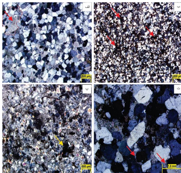
شکل ۴ الف) سیمان فراگیرنده که چند دانه را در بر گرفته است (پیکان قرمز رنگ). ب) سیمان هماتیته پیرامون دانه‌ها و پر کننده فضای خالی و زمینه سنگ (پیکان‌های قرمز رنگ). پ) سیمان هماتیته پرکننده شکستگی‌ها در یک رخساره ماسه‌سنگی متوسط دانه (پیکان‌های زرد رنگ). ت) جانشینی سیمان کلسیتی در دانه‌های چرتی و کوارتز. به خوردگی دانه‌های کوارتز توسط سیمان کلسیتی توجه شود (پیکان‌های قرمز رنگ).
