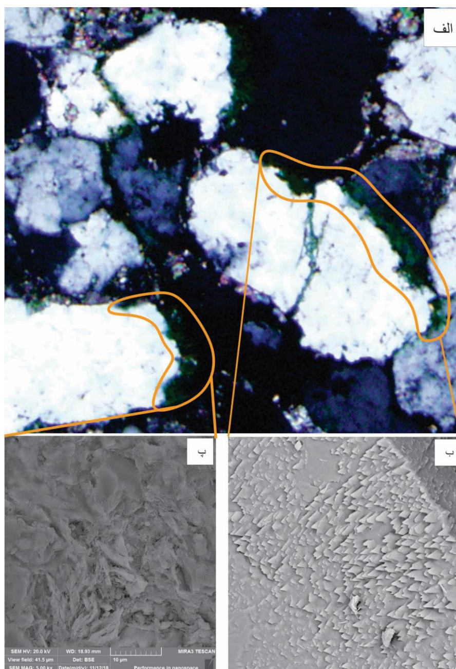
شکل ۷ تصاویر سنگ‌نگاری کانی رسی کلریت: (الف) تصویر میکروسکوپ نوری (XPL) کلریت با شکل پوشاننده ذرات که مانع از تشکیل سیمان کوارتزی و در نتیجه حفظ تخلخل و تراوایی می‌شود. (ب) تصویر میکروسکوپ الکترونی روبشی (SEM) کلریت با شکل بلورهای پولکی کوچک که سطح خارجی ذره‌ها را می‌پوشاند. (پ) تصویر میکروسکوپ الکترونی روبشی (SEM) کلریت با خاستگاه تخریبی.
