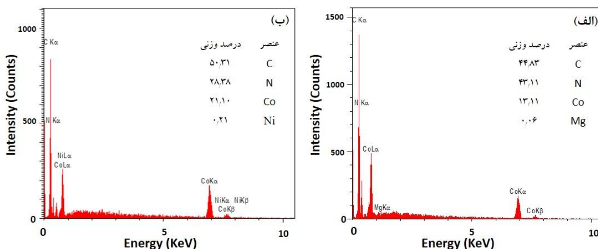
شکل ۴ طیف‌های پراکندگی انرژی پرتوی ایکس (EDX) از نمونه‌های (الف) MgCo-ZIF(150) و (ب) NiCo-ZIF(150).
