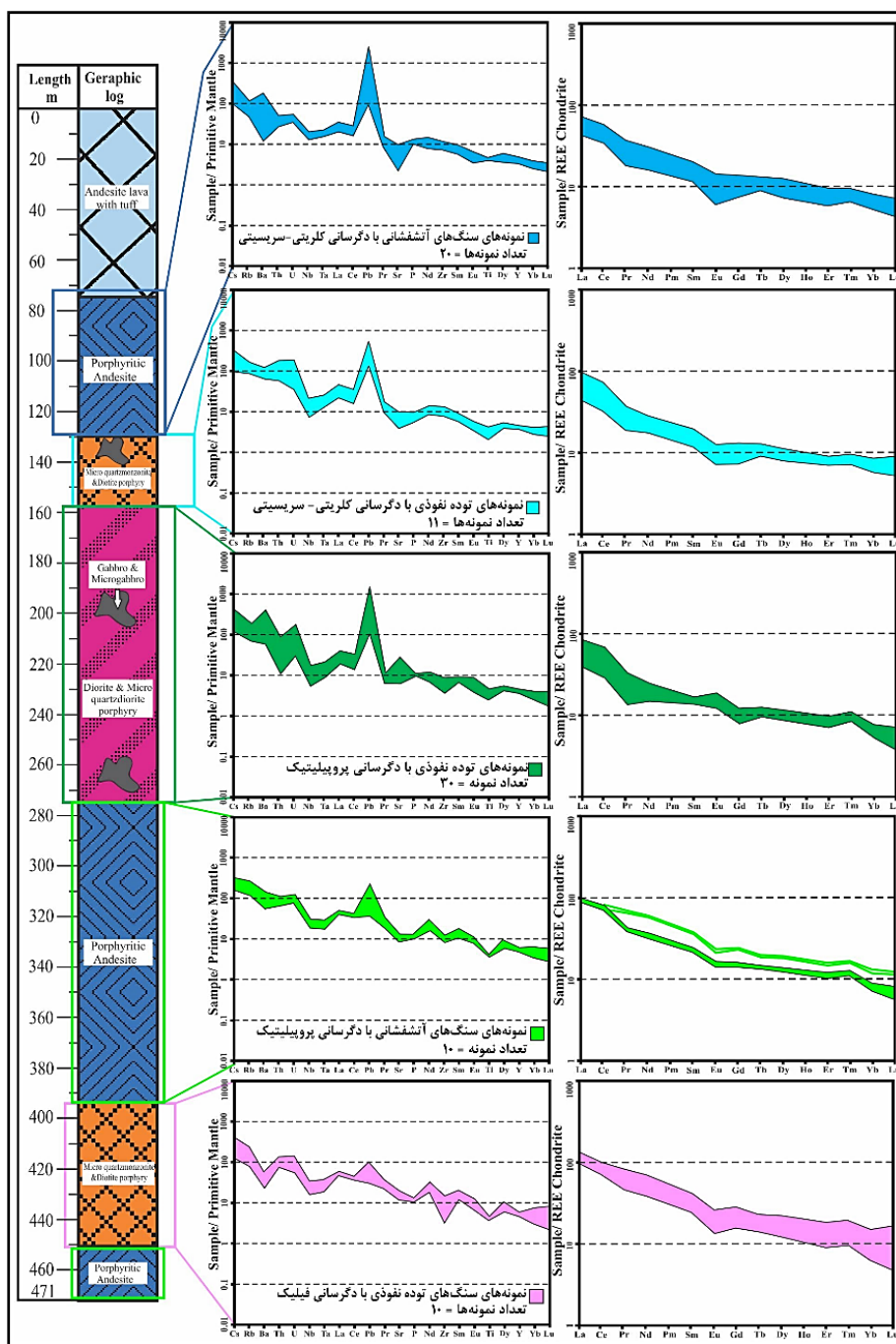
شکل ۱۱ روند تغییرات عمقی الگوی توزیع عناصر خاکی نادر بهنجار شده نسبت به کندریت [۴۴] و عناصر کمیاب بهنجار شده نسبت به گوشته اولیه [۴۵] در پهنه‌های دگرسانی کلریتی - سرسیتی، پروپیلیتی و فیلیک در توده نفوذی و واحد آندزیت پورفیری.
