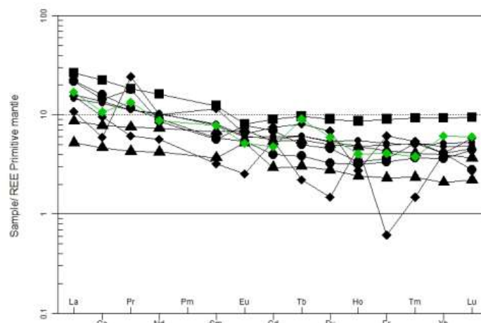
شکل ۹ نمودار غنکبوتی عناصر خاکی نادر بهنجار شده نسبت به کندریت [۹].
