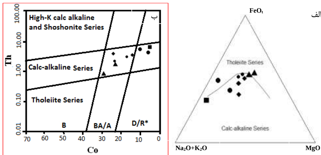
شکل ۶ الف) موقعیت نمونه‌های مورد بررسی بر الف) نمودار AFM [۵] و ب) نمودار Co نسبت به Th [۶] که همه نمونه‌ها به جز دو نمونه که به احتمال بسیار دگرسان شده‌اند در گستره سری آهکی قلیایی قرار دارند.
