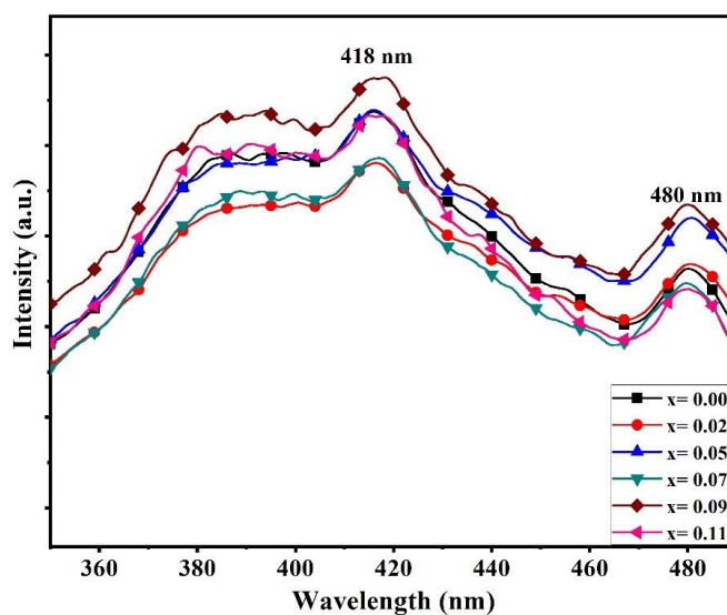
شکل ۱۰ طیف نورتایی نانوذرات \text{La}_{2-x}(\text{WO}_4)_3:\text{Gd}_x با غلظت‌های مختلف \text{Gd} (بر حسب میلی مول).
