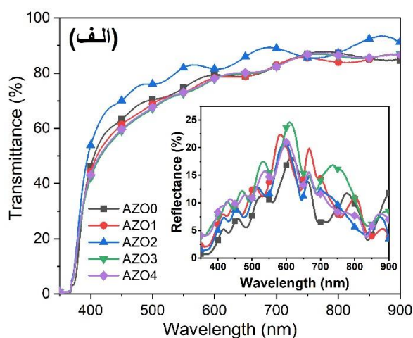
شکل ۵ الف) عبور و بازتاب نوری ب) نمودارهای تاؤک برای لایه‌های نازک AZO رشد یافته .
