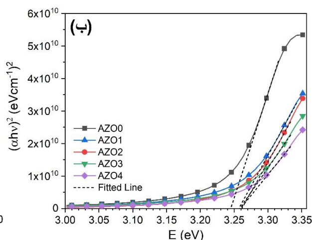
شکل ۵ الف) عبور و بازتاب نوری ب) نمودارهای تاؤک برای لایه‌های نازک AZO رشد یافته .
