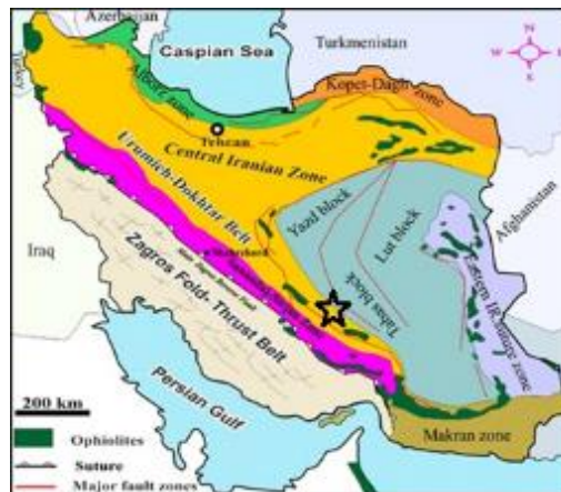
شکل ۱. موقعیت منطقه مورد بررسی در نقشه زمین‌شناسی واحدهای ساختمانی ایران [۱].
