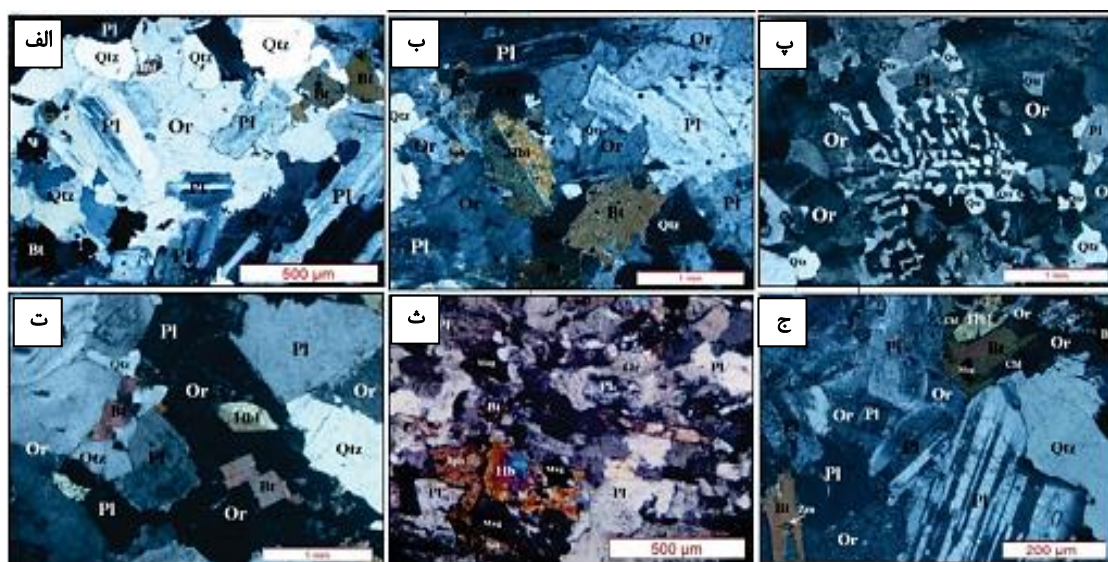
شکل ۴ تصاویر (XPL) از (الف) بافت گرانولار و بلورهای پلاژیوکلاز در توده علی‌آباد، (ب) بافت گرانولار و منشورهای هورنبلند در توده علی‌آباد، (پ) بافت میرمیکیتی و گرانوفیری در توده علی‌آباد، (ت) بافت گرانولار و حضور پلاژیوکلاز، ارتوکلازپریتی، هورنبلند، بیوتیت و کوارتز در توده نفوذی آدربلند، (ث) هورنبلند، بیوتیت، اسفن و اوپیک در توده آدربلند، (ج) درشت بلور پلاژیوکلاز، هورنبلند، بیوتیت و کلریت در توده نفوذی آدربلند.
