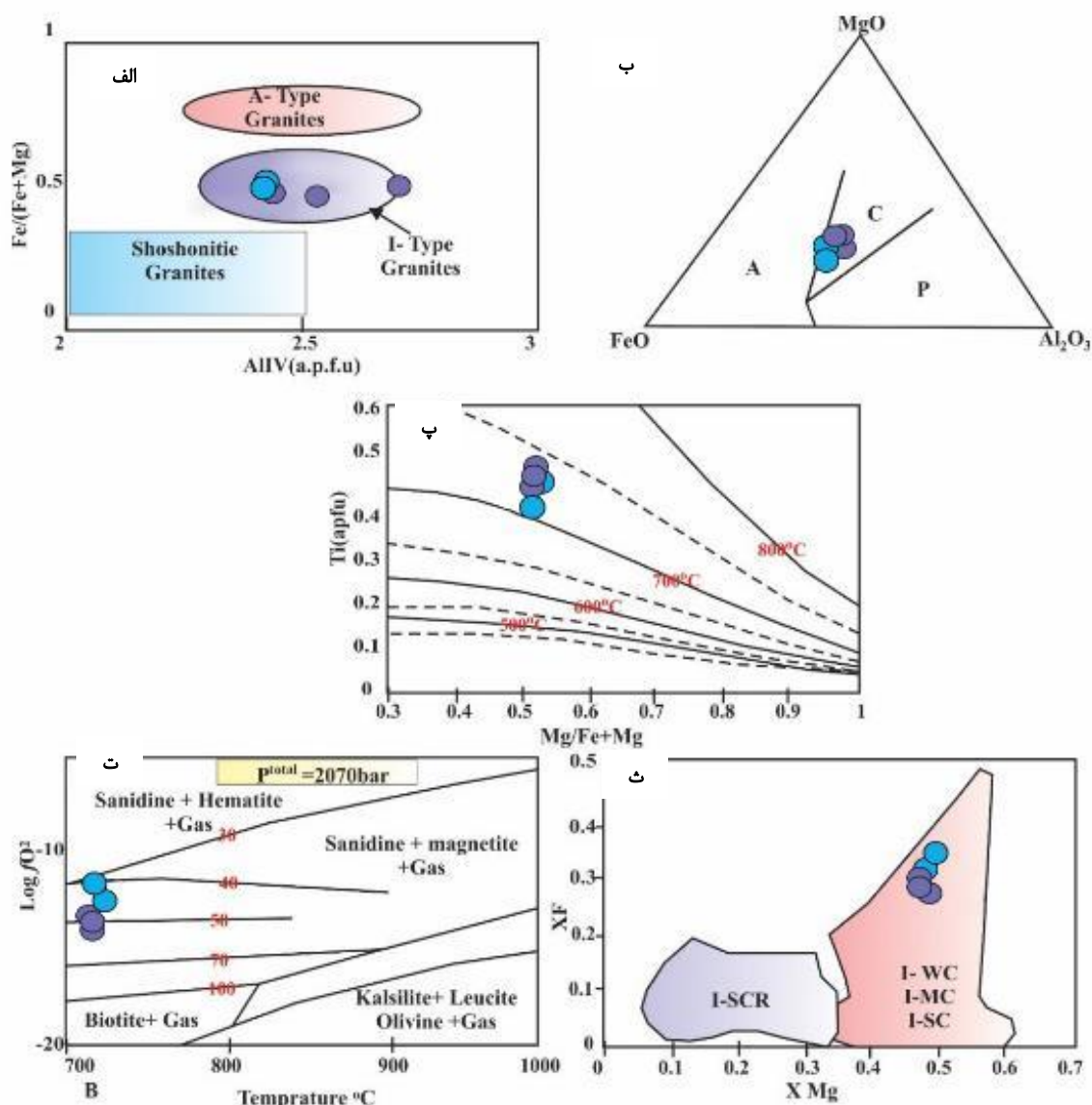
شکل ۱۰ الف) نمایش نمونه‌های بیوتیت در نمودار تغییرات Fe/(Fe+Mg) در مقابل AIV [۲۹]، ب) نمودار مثلثی FeO-MgO-Al_2O_3 در خصوص رده‌بندی تیپ سری‌ماگمای گرانیتوئیدی، پ) نمودار تعیین دما با استفاده از مقدار تیتان بیوتیت‌ها [۳۰]، ت) ترسیم نمونه‌ها در نمودار تغییرات Log fO_2 در مقابل دما بر حسب درجه سانتیگراد [۲۰]، ث) ترسیم بیوتیت‌های مورد بررسی در نمودارهای تخمین میزان آلودگی پوسته‌ای [۳۲].
