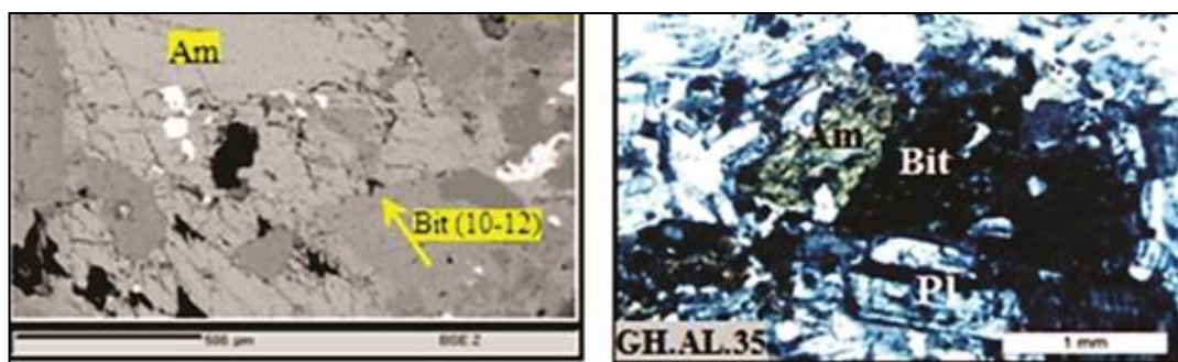
شکل ۸ تصاویر میکروسکوپی و الکترونی (BSE) از بیوتیت‌های همزیست با آمفیبول و پلاژیوکلاز در کوارتز دیوریت علی‌آباد.
