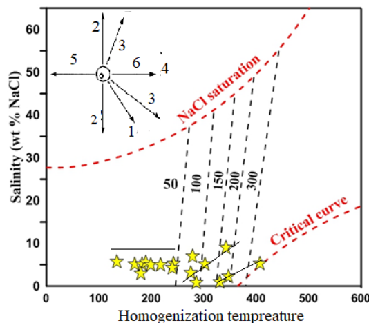
شکل ۱۰ همراه با روندهای تکامل سیال در بالایی سمت چپ [۲۳] و خطوط هم‌فشار در پایین [۳۲]. نمودار شوری نسبت به دمای هم‌گن‌شدگی که داده‌های منطقه مورد بررسی بیشتر در راستای افقی و فشار کمتر از ۳۰۰ بار واقع هستند.
