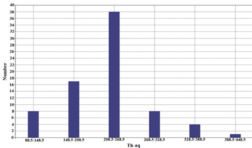
شکل ۹ نمودار ستونی دمای همگن‌شدگی میانبارهای سیال رگه- رگچه‌های کوارتزی شله‌بران.
