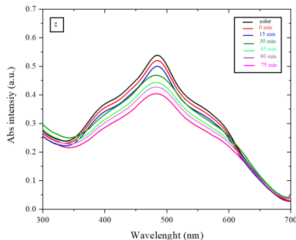
شکل ۸ بازده تخریب رنگ متیل قرمز برای فوتوکاتالیزور \text{Ag}_2\text{S}/\text{ZnS}/\text{Fe}_3\text{O}_4 زیر تابش نور فرابنفش در مدت ۷۵ دقیقه در (الف) \text{pH}=3 ، (ب) \text{pH}=7 و (پ) \text{pH}=9 .
