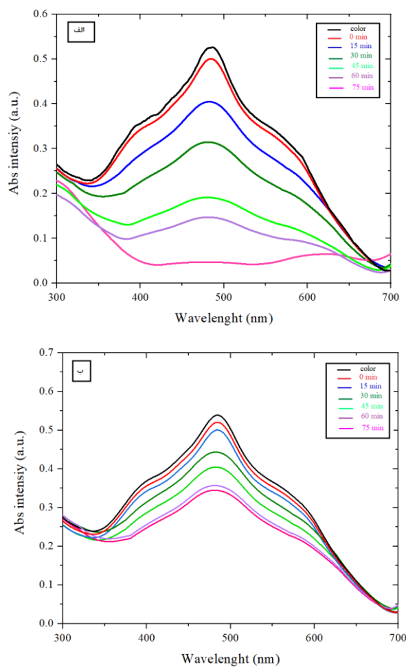
شکل ۷ بازده تخریب رنگ متیل قرمز برای فوتوکاتالیزورهای (الف) \text{Ag}_2\text{S}/\text{ZnS} و (ب) \text{Ag}_2\text{S}/\text{ZnS}/\text{Fe}_3\text{O}_4 زیر تابش نور مرئی در مدت ۷۵ دقیقه.
