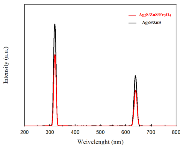
شکل ۴ طیف نوری نانوکامپوزیت های \text{Ag}_2\text{S}/\text{ZnS} و \text{Ag}_2\text{S}/\text{ZnS}/\text{Fe}_3\text{O}_4 .
