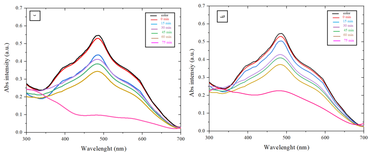
شکل ۷ بازده تخریب رنگ متیل قرمز برای فوتوکاتالیزورهای (الف) \text{Ag}_2\text{S}/\text{ZnS} و (ب) \text{Ag}_2\text{S}/\text{ZnS}/\text{Fe}_3\text{O}_4 زیر تابش نور مرئی در مدت ۷۵ دقیقه.
