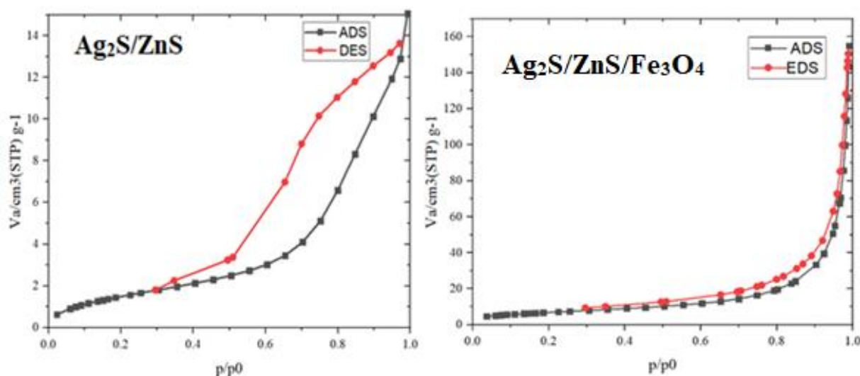
شکل ۵ منحنی های BET نانوکامپوزیت های \text{Ag}_2\text{S}/\text{ZnS} و \text{Ag}_2\text{S}/\text{ZnS}/\text{Fe}_3\text{O}_4 .
