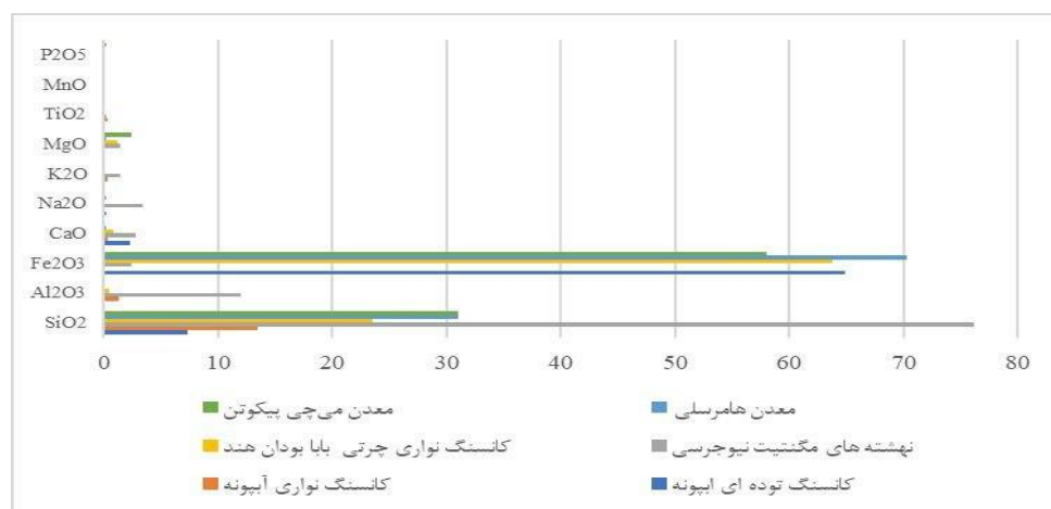
شکل ۱۵ نمودار چند عنصری برای مقایسه درصد اکسیدهای اصلی در کانسنگ‌های آیپونه با کانسنگ نیوجرسی [۲۹]، هامرسل [۳۰]، بابا بودان هند [۳۱]، می چی پیکتون [۳۲].
