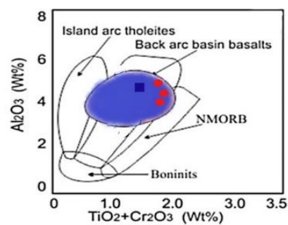
شکل ۴ الف نمودار Ti+Ca+Na؛ ب-نمودار Ti+Cr؛ پ-نمودار تعیین محیط زمین‌ساختی [۲۱] (VAB: بازالت های قوس آتشفشانی، WPA: بازالت‌های قلیایی درون صفحه‌ای، WPT: بازالت‌های تولیتی درون صفحه‌ای، OFB: بازالت‌های کف اقیانوسی، A: قلیایی، P: فوق قلیایی و S: نیمه قلیایی). ت- استفاده از کانی کلینوپیروکسن برای تعیین محیط زمین‌ساختی [۲۲]. ث- نمودار Al 2 O 3 به نسبت به TiO 2 +Cr 2 O 3 [۲۳] ج- نسبت Ca به Ti+Cr [۲۰].
