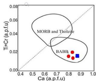
شکل ۴ الف نمودار Ti+Ca+Na؛ ب-نمودار Ti+Cr؛ پ-نمودار تعیین محیط زمین‌ساختی [۲۱] (VAB: بازالت های قوس آتشفشانی، WPA: بازالت‌های قلیایی درون صفحه‌ای، WPT: بازالت‌های تولیتی درون صفحه‌ای، OFB: بازالت‌های کف اقیانوسی، A: قلیایی، P: فوق قلیایی و S: نیمه قلیایی). ت- استفاده از کانی کلینوپیروکسن برای تعیین محیط زمین‌ساختی [۲۲]. ث- نمودار Al 2 O 3 به نسبت به TiO 2 +Cr 2 O 3 [۲۳] ج- نسبت Ca به Ti+Cr [۲۰].
