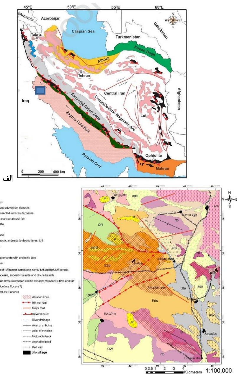
شکل ۱ الف- نقشه زمین‌شناسی ساده شده ایران [۱۱] بر اساس سن‌سنجی اورانیوم-سرب زیرکن سنگ‌های پرکامبرین ایران [۱۲]. ب- نقشه زمین‌شناسی منطقه مورد بررسی با کمی تغییر نسبت به نقشه زمین‌شناسی ابهر.
