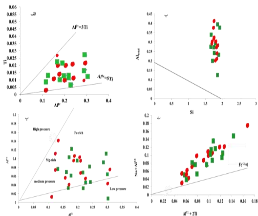
شکل ۷ (الف) نمودار Ti نسبت به Al^{IV} [۲۳]، (ب) نمودار Al نسبت به Si [۲۴] که نمونه‌های مورد بررسی در بالای خط اشباع جایگاه چاروچی قرار می‌گیرند، (پ) قرارگیری کلینوپیروکسن‌های حراران در منطقه کم فشار و فشار متوسط در نمودار Al^{IV} نسبت به Al^{VI} [۲۵] (ت) کلینوپیروکسن‌های اسکارن حراران در منطقه با گریزندگی زیاد در نمودار مرجع [۲۵] قرار می‌گیرند.
