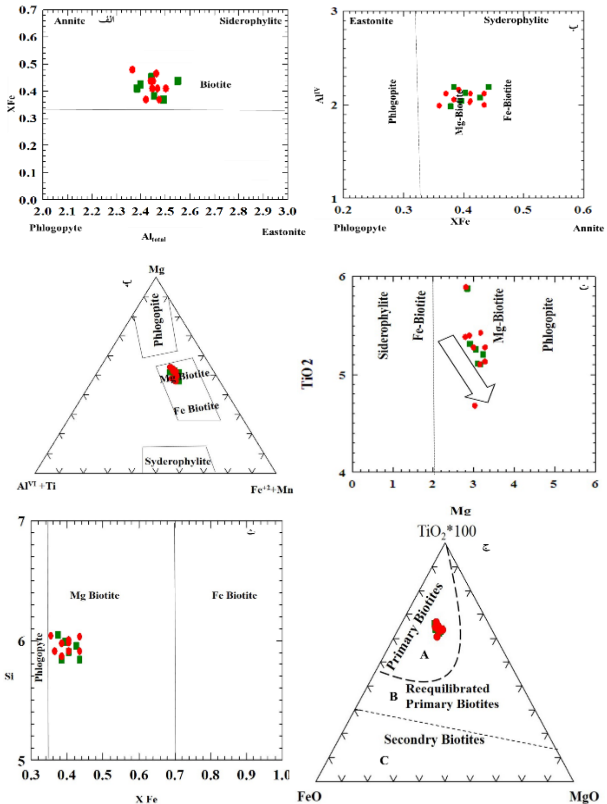
شکل ۳ الف تا ت رده‌بندی و ترکیب شیمیایی بیوتیت‌ها به ترتیب براساس نمودارهای X_{Fe} به نسبت Al^{IV} [۲۷]، Al^{IV} به نسبت X_{Fe} [۲]، نمودار سه‌تایی Mg-(Fe^{+2}+Mn)-(Al^{VI}+Ti) [۲۸]؛ نمودار TiO_2 نسبت به Mg [۲۹] و Si نسبت به X_{Fe} [۳۰] (ج) تعیین خاستگاه ماگما بر پایه مقدار TiO_2-FeO و MgO بیوتیت‌ها [۷].
