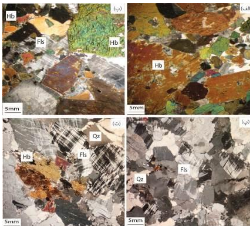
شکل ۳ تصاویر سنگ نگاری از سنگ‌های آبنیتی نقده: الف) هورنبلند نیمه شکل‌دار و درشت در سنگ آبنیتی مافیک، ب) هورنبلند های ریز تا درشت بلور همراه فلدسپارهای درشت در سنگ آبنیتی حدواسط، پ و ت) فلدسپار، میکروکلین با بافت مشبک و کوارتز و هورنبلند در سنگ گرانیتی.
