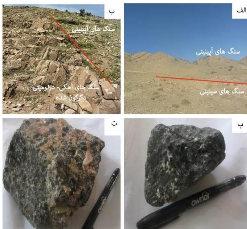
شکل ۲ تصاویر صحرایی سنگ‌های آبنیتی نقده: الف) بخشی از منطقه که سنگ‌های آبنیتی و گرانیت با مرز گسلی دیده می‌شوند، ب) مرز برخورد توده آبنیتی و سنگ‌های آهکی و دولومیتی دگرگون شده به سن کرتاسه [۱۸]، پ و ت) نمونه دستی از سنگ‌های مافیک-حدواسط آبنیتی نقده.
