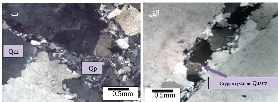
شکل ۱۲ انواع مختلف کوارتز در مقاطع موردبررسی در XPL. الف) کوارتز نهان بلور. ب) کوارتز تک بلور (Qm) بسیلور (Qp).
