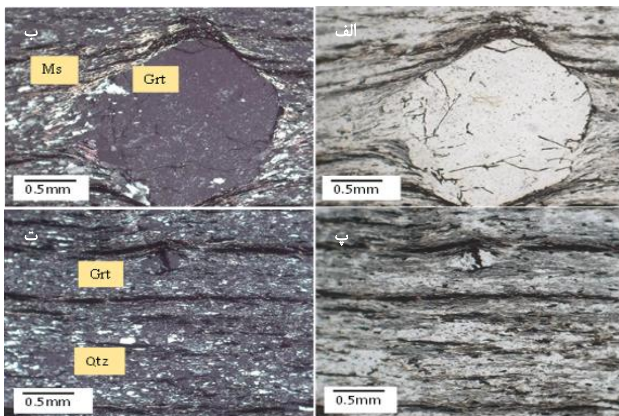
شکل ۷ تصاویر میکروسکوپی از گارنت میکاشیست: الف) بلور گارنت پیش از اعمال نیروهای زمین‌ساختی (PPL، همان عکس در XPL، پ) بلور گارنت هم‌زمان با اعمال نیروهای زمین‌ساختی (XPL، ت) همان عکس در PPL. (Grt: گارنت، Ms: مسکوویت، Qtz: کوارتز [۱۸]).
