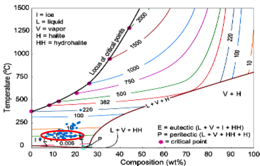
شکل ۱۶ تعیین فشار سیال در کانی کوارتز منطقه مورد بررسی بر اساس نمودار اتکینسون [۳۹].
