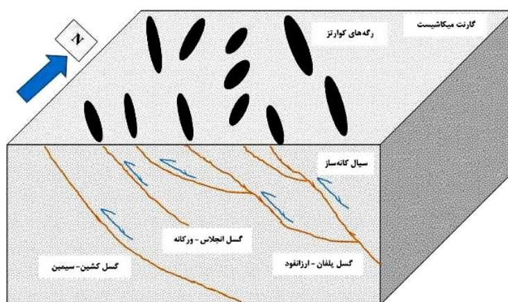
شکل ۲۱ طرحواره پیشنهادی برای تشکیل رگه‌های کوارتز در منطقه ارزانفود.
