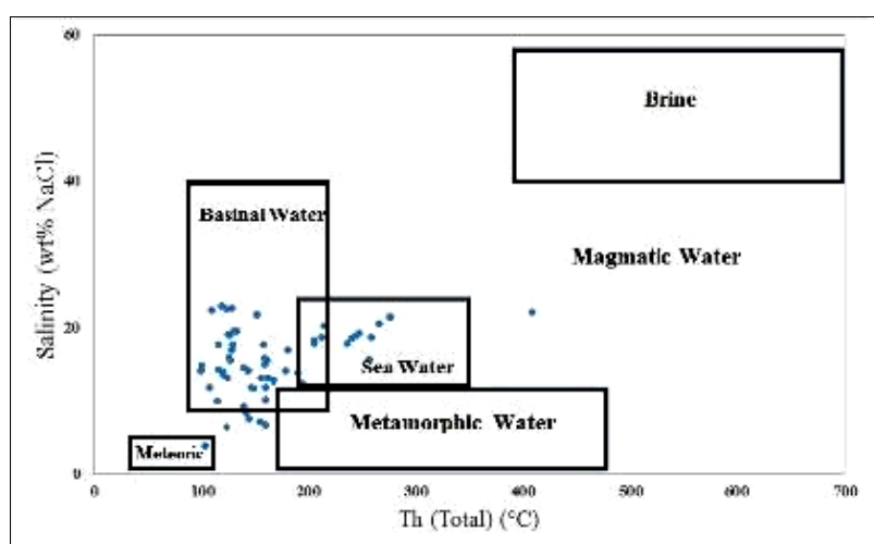
شکل ۲۰ نمودار شوری- دمای همگن‌شدگی برای تعیین خاستگاه سیال‌های منطقه ارزانفود [۴۱].
