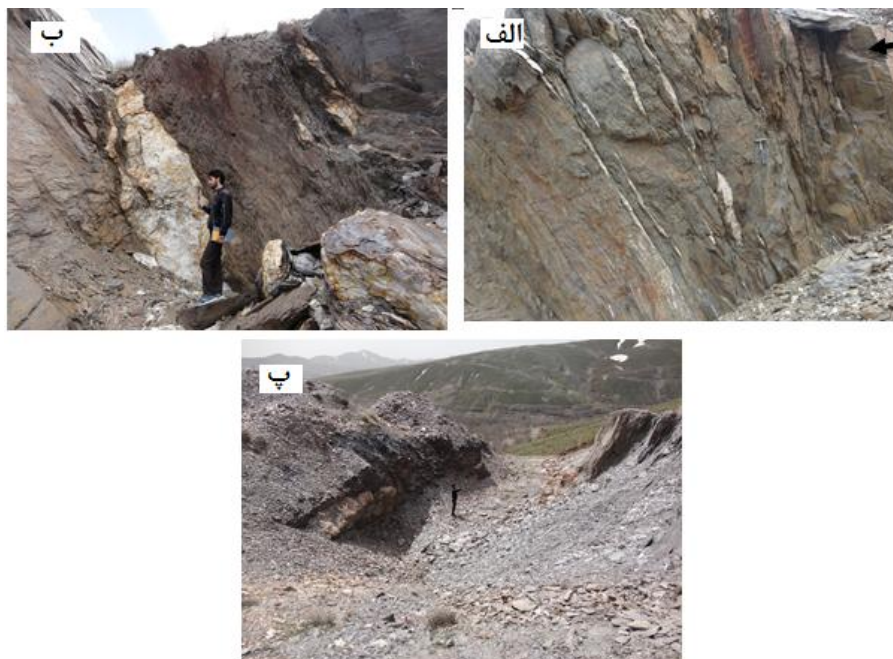
شکل ۵ انواع رگه‌های کوارتز در منطقه مورد بررسی: الف) رگه‌های نوع ۱ در راستای درزه‌های منطقه. ب) رگه‌های نوع ۲ و پ) رگه‌های نوع ۳.
