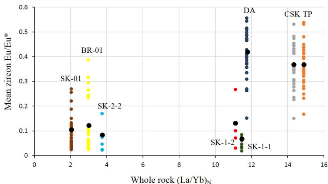
شکل ۴ میانگین ناهنجاری Eu/Eu^* زیرکن نسبت به (La/Yb)_N سنگ کل بهنجار شده به کندریت [۲۹]. خطا براساس ۲ سیگما محاسبه شده است.
