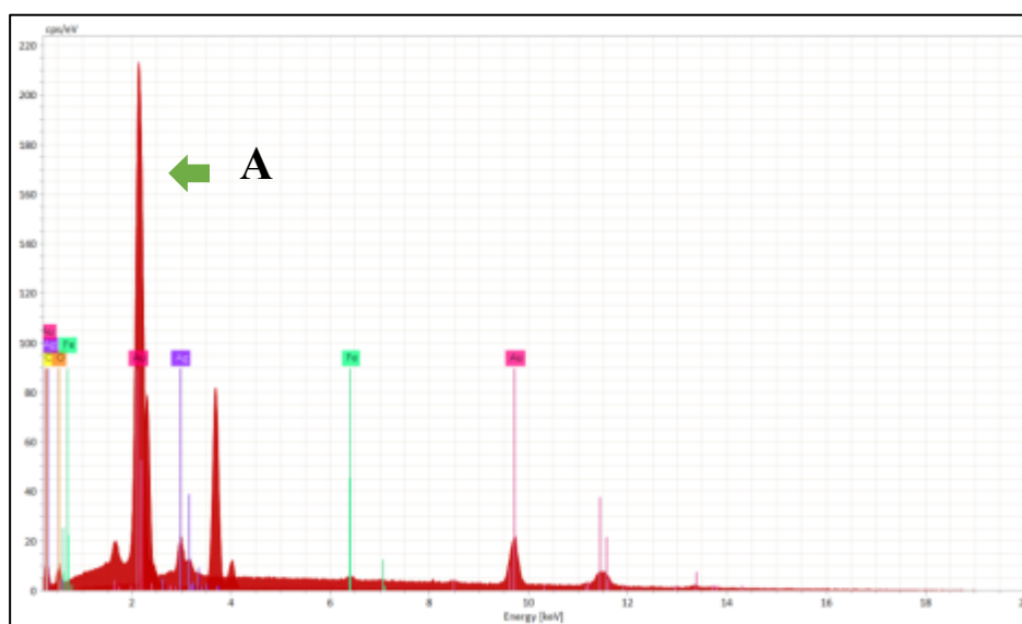
شکل ۷ تصویر SEM با بزرگنمایی ۳۶۴۰ از دانه های الکتروم که به صورت سفید و زاویه دار درون لیمونیت قرار دارند و اندازه دانه ۳/۸ تا ۴ میکرومتر است. طیف تجزیه نقطه ای از بخش طلا دار گرفته شده است که بالاترین قله مربوط به طلاست.
