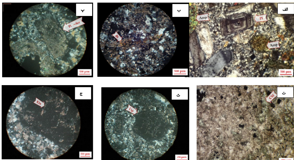
شکل ۴ الف) تصویر میکروسکوپی از توده پورفیری شادان با بافت پورفیری و زمینه ریزدانه‌ای و درشت بلورهای آمفیبول و پلاژیوکلاز، ب) حضور بیوتیت ثانویه همراه با کانی‌های کدر (به صورت رگچه) در اثر دگرسانی پتاسیمی در توده پورفیری شادان، پ) دگرسانی فلیک و تبدیل تقریباً کامل درشت بلورهای پلاژیوکلاز و فلدسپار پتاسیمی به سریسیت و پاراگونیت، ت) تصویر میکروسکوپی از دگرسانی پروپلیتیک در سنگ‌های توفی با حضور کلریت، ث و ج) تبدیل فلدسپار به کانی‌های رسی. همه تصاویر در نور قطبیده متقاطع (XPL) تهیه شده‌اند. (آمفیبول: Amp، بیوتیت: Bt، پلاژیوکلاز: Pl، سریسیت: Ser، کوآرتز: Qz، فلدسپار: Fsp، کائولینیت: Kln، کلریت: Chl).
