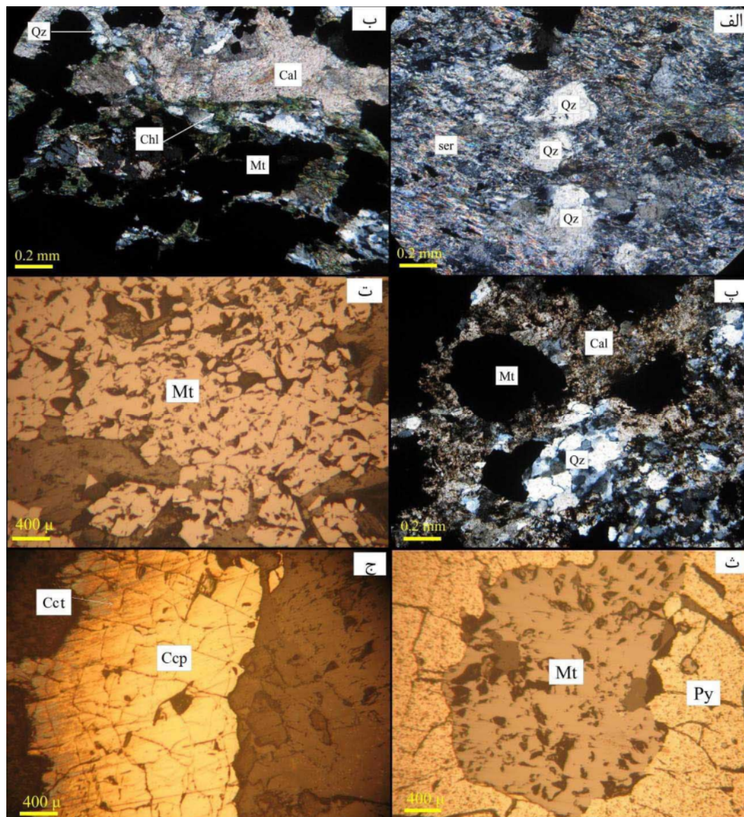
شکل ۳ تصاویر میکروسکوپی سنگ میزبان و کانسنگ آهن بالستان: الف) سنگ میزبان کوارتز-سربیسیت شیبست بدون کانه‌زایی که جهت یافتگی کوارتز و سربیسیت در آن قابل مشاهده است (نور قطبیده متقاطع، xpl)، ب) کلسیت، کوارتز و کلریت همراه با کانه‌زایی (نور xpl)، پ) کلسیت و کوارتز برآمده از دگرگونی و همراه با کانه‌زایی (نور xpl)، ت) مگنتیت (نور بازتابی)، ث) مگنتیت به همراه پیریت (نور بازتابی)، ج) کالکوپیریت که از لبه و در راستای سطوح رخ به کالکوسیت تبدیل شده است (نور بازتابی). کوارتز: Qz، کلسیت: Cal، کلریت: Chl، سربیسیت: Ser، مگنتیت: Mt، پیریت: Py، کالکوپیریت: Ccp، کالکوسیت: Cet [۳].
