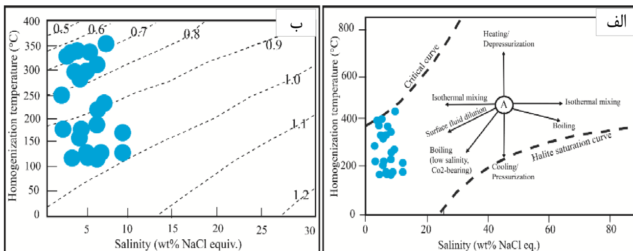
شکل ۱۰ الف) نمودار دمای همگن‌شدگی مایع-گاز سیال‌های درگیر کانسار نسبت به شوری در سامانه \text{NaCl-H}_2\text{O} [۲۰] و ب) نمودار شوری-دما برای محاسبه چگالی سیال‌های درگیر [۲۱].
