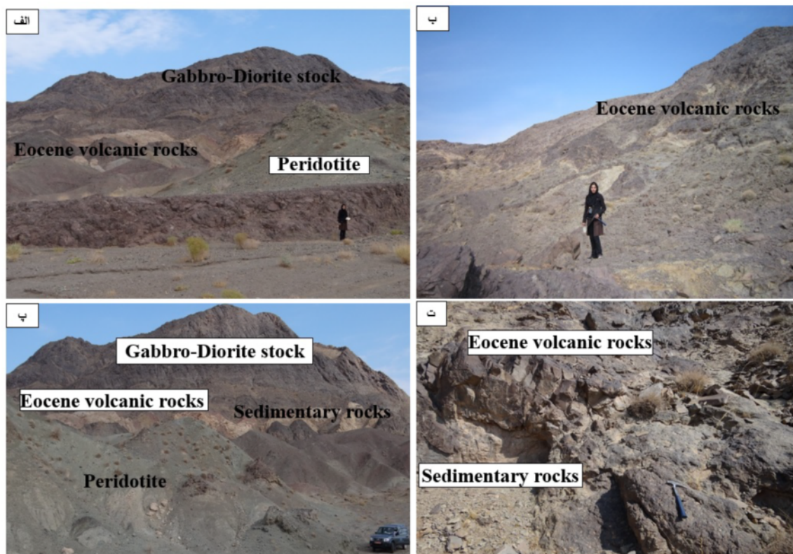
شکل ۲ تصاویر صحرایی منطقه کلوت قندهاری: الف- سنگ‌های آتشفشانی ائوسن به همراه استوک گابرویی- دیوریتی و واحدهای پریدوتیتی، ب- نمایی از سنگ‌های آتشفشانی ائوسن کوه کلوت قندهاری، پ- سنگ‌های آتشفشانی ائوسن به همراه استوک گابرویی- دیوریتی، واحدهای رسوبی و پریدوتیت و ت) سنگ‌های آتشفشانی ائوسن به همراه واحدهای رسوبی.
