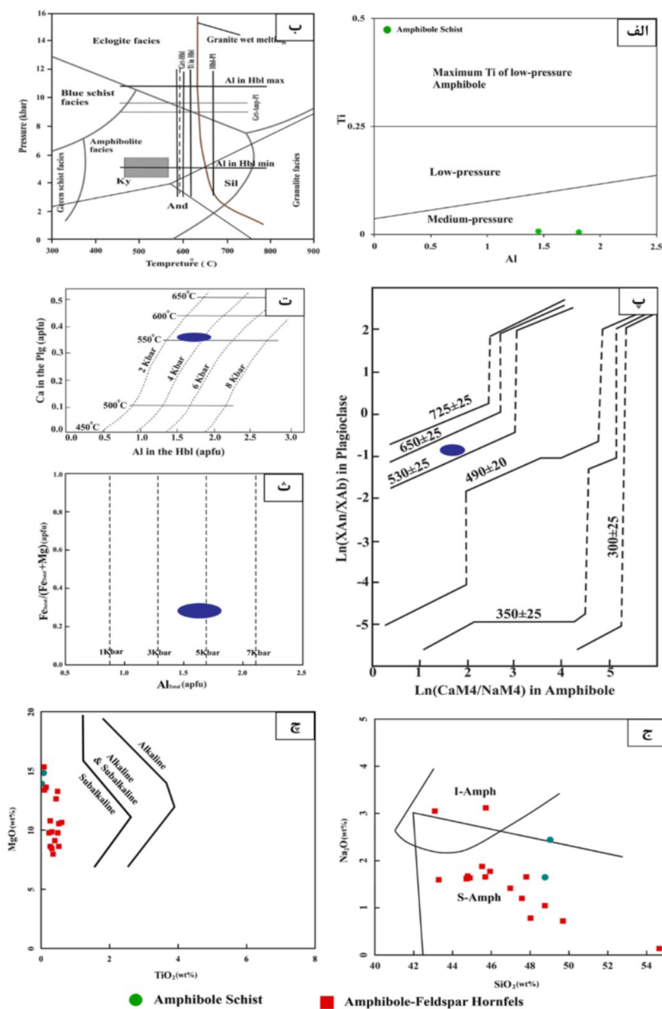
شکل ۷ الف) نمودار Ti نسبت به Al [۳۲] که بر اساس آن، آمفیبول شلیست‌ها در فشارهای متوسط تشکیل شده‌اند، ب) دما و فشار تشکیل سنگ های دگرگونی منطقه گرمخانی-میهم، گستره رخساره برگرفته از مرجع [۴۷] است، پ) بررسی دمای دگرگونی آمفیبول شلیست‌ها با استفاده از نمودار \text{Ln}(\text{XAn}/\text{XAb}) در پلاژیوکلاز نسبت به \text{Ln}(\text{CaM4}/\text{NaM4}) [۴۳]، که نمونه‌های مورد بررسی در گستره دمایی ۵۵۰-۵۳۰±۲۵ درجه سانتی‌گراد قرار دارند، ت) تعیین همزمان دما و فشار در نمودار Ca پلاژیوکلاز نسبت به Al آمفیبول [۲۸] که دما و فشار به ترتیب ۵۵۰-۵۶۰ درجه سانتی‌گراد و ۳-۵ کیلو بار را نشان می‌دهد، ث) در نمودار \text{Al}_{\text{Total}}/(\text{Fe}_{\text{Total}}+\text{Mg}) نسبت به \text{Fe}_{\text{Total}} [۳۳] که براساس آن، نمونه‌های مورد بررسی در گستره فشار ۴-۶ کیلو بار قرار دارند، ج) نمودار رده‌بندی زمین‌ساختی ماگمایی آمفیبول‌ها [۴۸] که بیانگر تشکیل آمفیبول‌های مورد بررسی در محیط‌های وابسته به ابرفرورانشی است، چ) نمودار بررسی قلیایی و شبه‌قلیایی بودن آمفیبول‌ها [۴۹] که بر اساس آن، آمفیبول‌های مورد بررسی ماهیت شبه قلیایی دارند، (آمفیبول‌های ابرفرورانشی)، (آمفیبول‌های درون صفحه‌ای).
