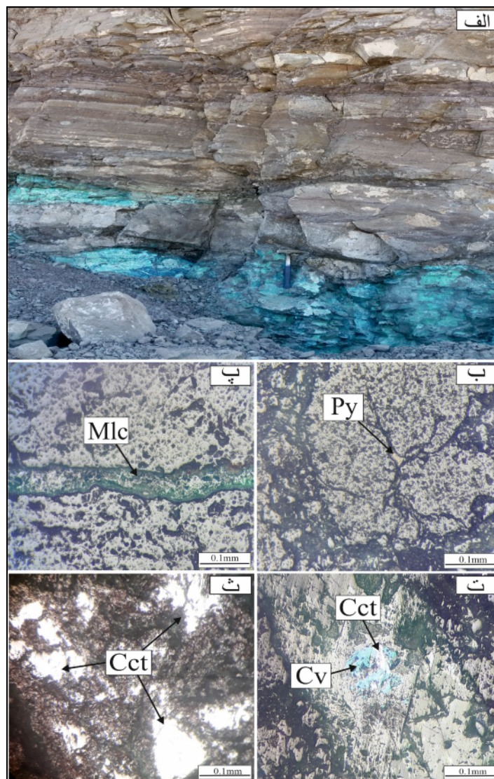
شکل ۶ الف) تصویر صحرایی از کانی‌سازی به شکل عدسی و هم‌روند با سنگ میزبان ماسه‌سنگی، ب) کانی پیریت با بافت پراکنده، پ) رگچه مالاکیت، کالکوسیت و کوولیت، ت) کالکوسیت و کوولیت و ث) کالکوسیت اولیه. (Py= پیریت، Mlc= مالاکیت، Cct= کالکوسیت، Cv= کوولیت [۱۵].
