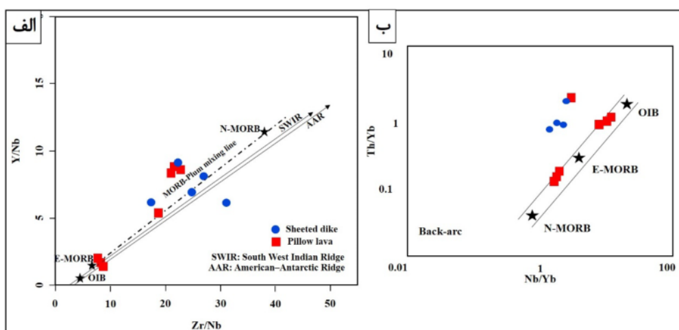
شکل ۱۳ موقعیت نمونه‌های مورد بررسی در آمیزه افیولیتی دومک بر (الف) نمودار Y/Nb نسبت به Zr/Nb و (ب) نمودار Th/Yb نسبت به Nb/Yb [۴۰]، (داده‌های N-MORB, E-MORB و OIB برگرفته از مرجع [۳۱]، داده‌های SWIR برگرفته از مرجع [۴۱] و داده‌های AAR برگرفته از مرجع [۴۲]).
