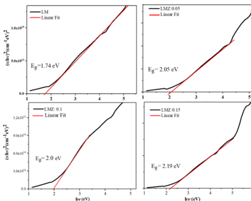
شکل ۴ منحنی (\alpha h\nu)^2 نسبت به h\nu برای نمونه‌های \text{LaMn}_{1-x}\text{Zn}_x\text{O}_3 ( x=0, 0.05, 0.1, 0.15 ).
