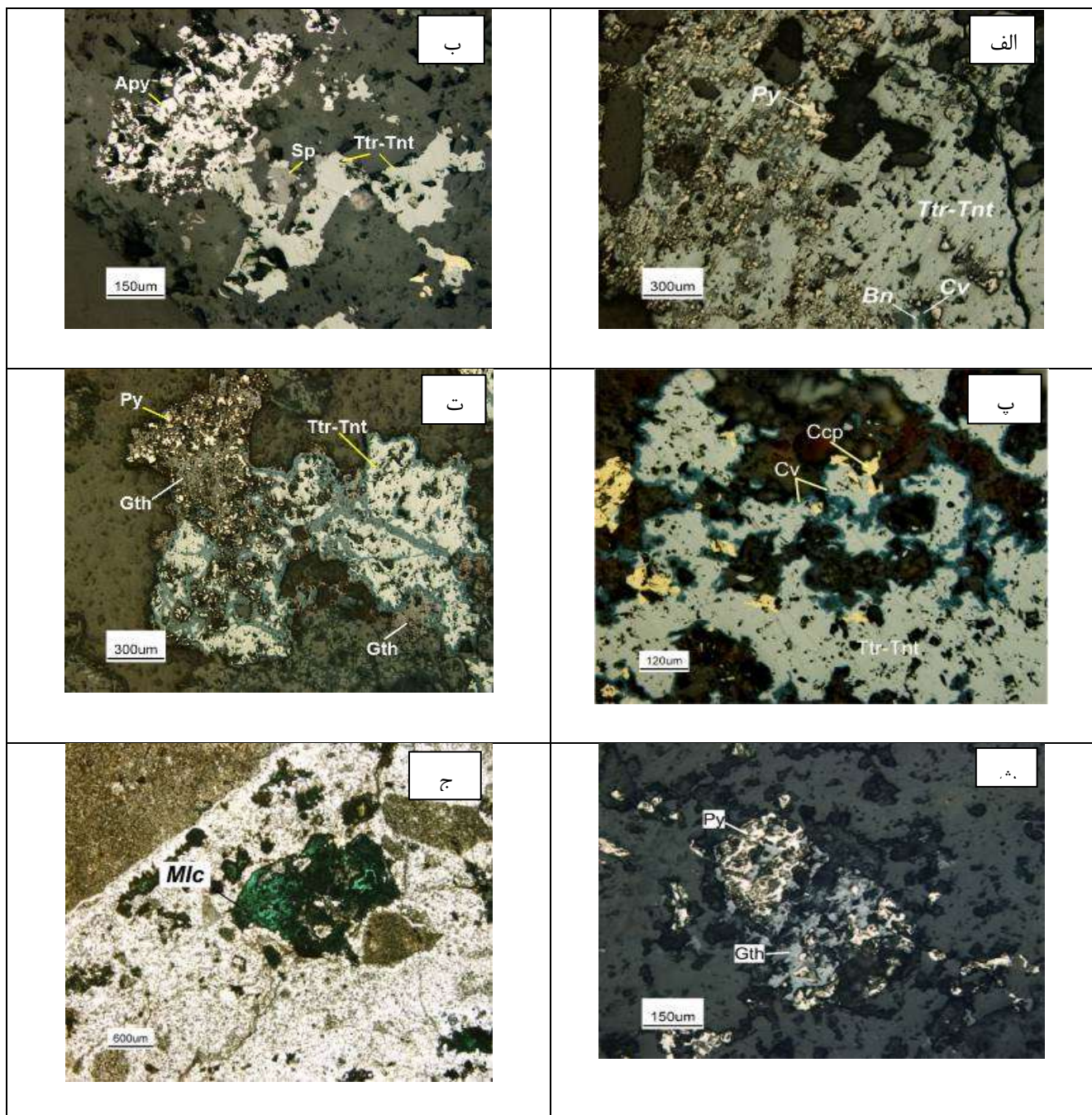
شکل ۵ تصاویر میکروسکوپی از کانی‌های مختلف تشکیل دهنده کانسنگ: (الف) جانشینی پیریت (Py) افشان با تتراهدریت-تنانتیت (Ttr-Tnt) در PPL، (ب) جانشینی سری تتراهدریت-تنانتیت (Ttr-Tnt) با آرسنوپیریت (Apy) در PPL، (پ) کوولیت (Cv) بصورت لایه‌ای نازک جانشین تتراهدریت-تنانتیت (Ttr-Tnt) شده است (PPL)، (ت) کانی‌سازی پیریت (Py) به صورت پراکنده در متن سنگ که به گوتیت (Gth) دگرسان شده است (PPL؛ ث) رخداد پیریت (Py) و گوتیت (Gth) در سنگ (PPL)؛ و (ج) پرشدن حفره‌های سنگ با مالاکیت (Mlc) در PPL.
