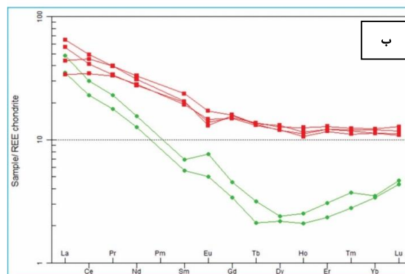
شکل ۷ الف- نمودار عنکبوتی بهنجار شده با گوشته اولیه [۱۹] برای عناصر خاکی نادر و برخی از عناصر کمیاب؛ و ب- نمودار عنکبوتی عناصر خاکی نادر بهنجار شده با کندریت [۱۸].
