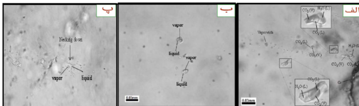
شکل ۶ انواع سیال‌های درگیر دیده شده در نمونه‌های کوارتز منطقه مورد بررسی: الف) سه فازی (H 2 O-CO 2 -NaCl) (ب) دو فازی (LCO 2 +VH 2 O ، VH 2 O+LH 2 O ، LCO 2 +VCO 2 ) (پ) پدیده دم بریدگی.
