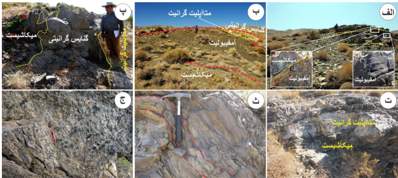
شکل ۲ رخمون آمفیبولیت و میکاشیست در زیرپهنه مرکزی: الف) میان‌لایه آمفیبولیت در میکاشیست‌ها، ب) گنیس گرانیتی و متاآلیت-گرانیت در همبری با آمفیبولیت و میکاشیست، پ) همبری متاآلیت-گرانیت، گنیس گرانیتی و میکاشیست، ت) میکاشیست و نفوذ متاآلیت-گرانیت در آن، ث) چین‌خوردگی و برگوارگی در میکاشیست و ج) درشت بلورهای گارنت در گارنت-میکاشیست.
