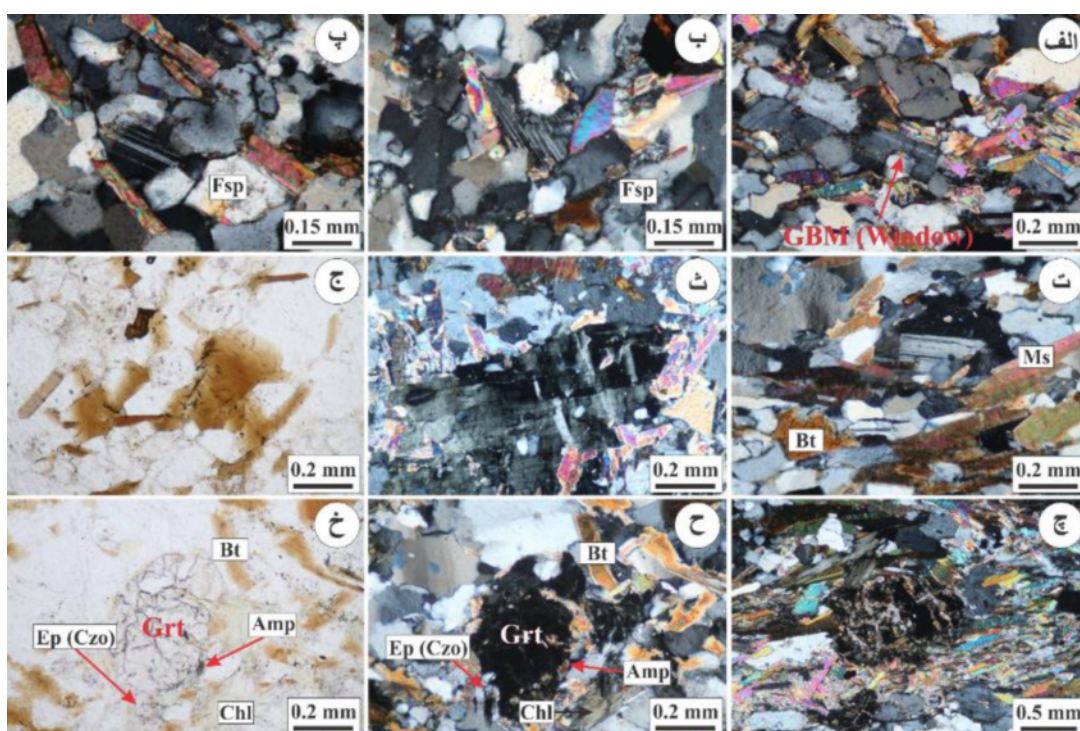
شکل ۵ الف) مهاجرت مرز دانه‌ای (GBM) در کانی پلاژیوکلاز (XPL). ب و پ) ماکل دگرشکلی نوک تیز شده در کانی پلاژیوکلاز و حضور فلدسپات‌های سریسیتی شده (XPL). ت) ماکل‌های دگرشکلی و خاموشی موجی در کانی پلاژیوکلاز (XPL). ث) نوارهای دگرشکلی پیچ‌خورده در کانی کلریت (XPL). ج) بافت ساژنیتی دربردارنده سوزن‌های روتیل در کانی بیوتیت (PPL). چ) حضور مسکویت فنژیستی و گارنت دارای شکستگی‌های متقاطع و کششی عمود بر برگواره (XPL). ح و خ) کانی گارنت در حال تجزیه به آمفیبول و اپیدوت بترتیب در XPL و PPL. (Fsp = فلدسپار، Ms = مسکویت، Bt = بیوتیت، Grt = گارنت، Amp = آمفیبول، Ep = اپیدوت، Czo = کلینوزوئیزیت، Chl = کلریت).
