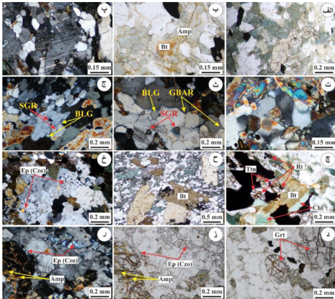
شکل ۶ الف) بلورهای آمفیبول در مقطع عرضی با دو دسته رخ متقاطع (PPL). ب) بیوتیت در حال نقش بستن بر بلورهای آمفیبول (PPL). پ) پلاژیوکلاز با ماکل دگرشکلی خمیده و نوک تیز و سریستی شدن در راستای ماکل‌ها (XPL). ت) ماکل دگرشکلی نوک تیز شده در پلاژیوکلاز (XPL). ث) بافت دگرشکلی برآمدگی مرز دانه، چرخش ریزدانه و مرزهای چندگوشی با زاویه 120^\circ برای کانی کوارتز و فلدسپات‌های سریستی شده (XPL). ج) بافت دگرشکلی برآمدگی مرز دانه و چرخش ریزدانه در کانی کوارتز (XPL). چ) بلورهای روتیل درحال تجزیه به ایلمنیت و تیتانیت و کانی بیوتیت درحال کلریتی شدن (XPL). ح) درشت بلور بیوتیت که از جهت‌یافتگی اصلی سنگ پیروی نمی‌کند (XPL). خ) حضور کلینوزوئیزیت بصورت میانبار در پلاژیوکلاز (XPL). د) بلور گارنت دارای شکستگی‌های متقاطع و عمود بر برگواره (PPL). ذ و ر) درشت بلور گارنت درحال تجزیه به اپیدوت (کلینوزوئیزیت) و آمفیبول به ترتیب در PPL و XPL. Amp: آمفیبول، Bt: بیوتیت، Rt: روتیل، Ttn: تیتانیت، Chl: کلریت، Ep: اپیدوت، Czo: کلینوزوئیزیت، Grt: گارنت.
