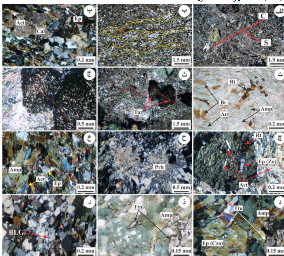
شکل ۸ الف) بافت‌های ورقه شکفتی و دگرشکلی S-C در آمفیبول-شیست (XPL). ب) برگواره شاخه‌ای در آمفیبول-شیست‌ها (XPL). پ) کانی‌های اپیدوت، کلسیت و اکتینولیت در آمفیبول-شیست (XPL). ت) بلورهای آمفیبول و اکتینولیت در حال بیوتیتی شدن (PPL). ث و ج) درشت‌بلور تورمالین دارای میانبراهایی هم راستا با برگواره آمفیبول-شیست‌ها (XPL). چ) میانبراهای زوئیزیت، روتیل و اکتینولیت در درشت‌بلور تورمالین. ح) بلورهای پرنهیت پرکننده حفره‌ها و شکستگی‌ها (XPL). خ) بلورهای اپیدوت، اکتینولیت و آمفیبول در آمفیبولیت (XPL). د و ذ) بلورهای لوزی رخ تیتانیت و آمفیبول‌های در حال بیوتیتی شدن در آمفیبولیت‌ها (بترتیب در XPL و PPL). ر) ریزساختار دگرشکلی برآمدگی مرز دانه در کانی کوارتز (XPL). Cal=کلسیت، Ep=اپیدوت، Act=اکتینولیت، Bt=بیوتیت، Amp=آمفیبول، Tur=تورمالین، Rt=روتیل، Czo=Czo=کلینوزوئیزیت، Act=اکتینولیت، Prh=پرنهیت، Ttn=تیتانیت).
