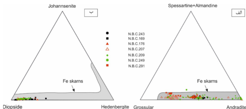
شکل ۱۲ الف- ترکیب گارنت‌های مورد بررسی در نمودار سه‌تایی گارنت‌ها و مقایسه آن‌ها با گارنت‌های همراه با اسکارن‌های آهن و ب- ترکیب پیروکسن‌های مورد بررسی در نمودار سه‌تایی هدنبرژیت-دیوپسید-ژوهانسنیت و مقایسه آن‌ها با پیروکسن‌های همراه با اسکارن‌های آهن [۳۲].
