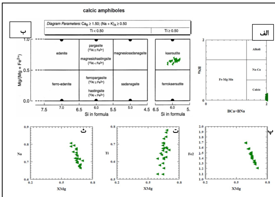
شکل ۵ ترکیب آمفیبول در گابروی قلیایی مونزو گابرو: الف) نمودار BNa-BNa+BCa که براساس آن، نمونه‌ها در گستره آمفیبول‌های کلسیمی قرار دارد. ب) در نمودار MgMg+Fe 2+ -Si که براساس آن و با توجه به Ti > 0.5 نمونه از نوع کرسوتیت است. پ، ت و ث) تغییرات عناصر Fe 2+ ، Na و Ti نسبت به Mg #
