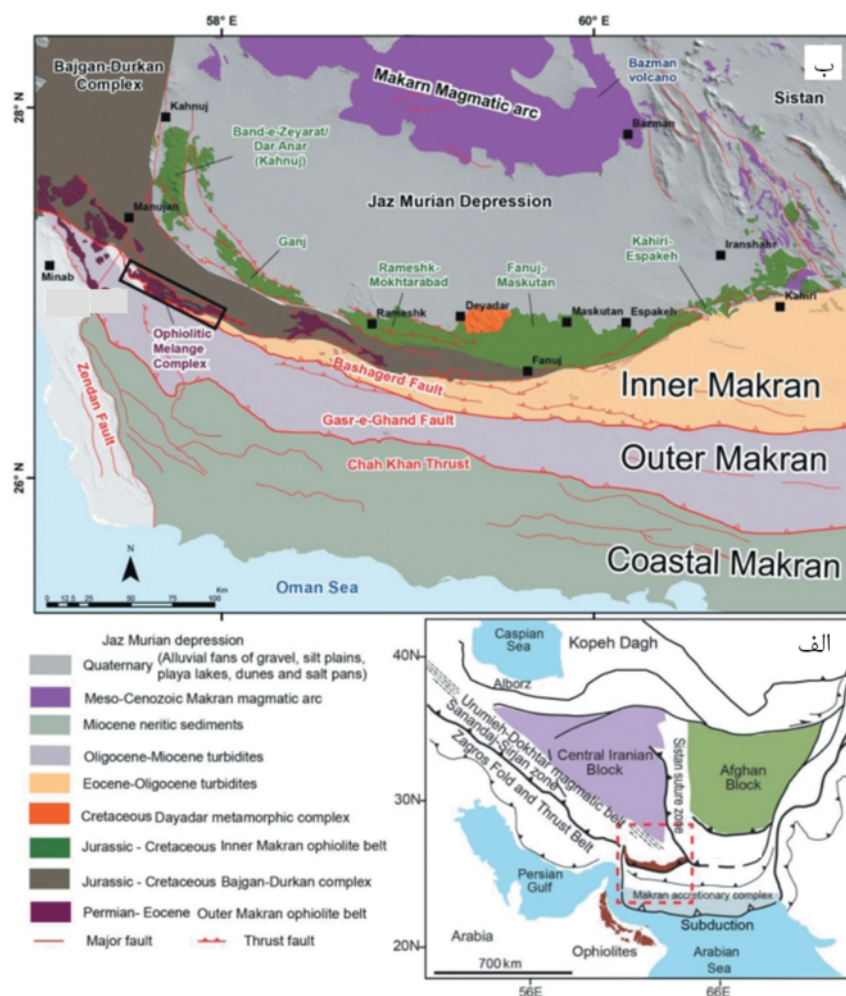
شکل ۱ الف) نقشه‌ی زمین‌ساختی ایران با تاکید بر واحدهای زمین‌ساختی ماگمایی، ب) موقعیت کلی و ساده شده‌ای از واحدهای ساختاری سنگ زمین‌ساختی منشور برفازایشی مکران [۸].
