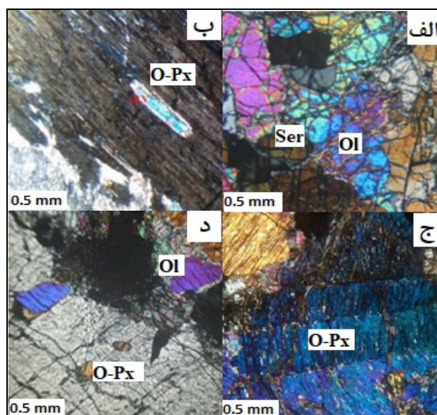
شکل ۷ مقاطع میکروسکوپی نازک از کانسار چشمه بید: الف) الیوین و پدیده سرپانتینی شدن در محل شکستگی و رخ‌های کانی در کانسار چشمه بید، ب) کانی ارتوپیروکسن، پ) بافت شکنجی در ارتوپیروکسن‌ها و ت) میانبارهای الیوین درون کانی ارتوپیروکسن. (Ol: الیوین، O-Px: ارتوپیروکسن و Ser: سرپانتین).
