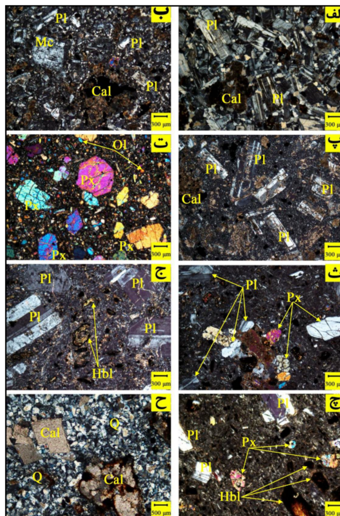
شکل ۴ تصویر میکروسکوپی در نور قطبیده متقاطع (XPL): الف) دیوریت پورفیری (حضور درشت بلورهای پلاژیوکلاز در زمینه ریزدانه)، ب) مونزودیوریت پورفیری (دگرسانی پلاژیوکلازها به سریسیست و کربنات)، پ) آندزیت (بلورهای پلاژیوکلاز در زمینه شیشه‌ای)، ت) بازالت (کانی پیروکسن در زمینه ریزدانه و شیشه‌ای)، ث) پیروکسن آندزیت (حضور پلاژیوکلاز و پیروکسن در زمینه ریزدانه)، ج) هورنبلند آندزیت (حضور هورنبلند در زمینه ریزدانه)، چ) هورنبلند پیروکسن آندزیت (حضور پلاژیوکلاز، پیروکسن و هورنبلند در زمینه دانه ریز) و ح) رگه سیلیسی - برشی، نشانه‌های اختصاری برگرفته از مرجع [۱۵] هستند.
