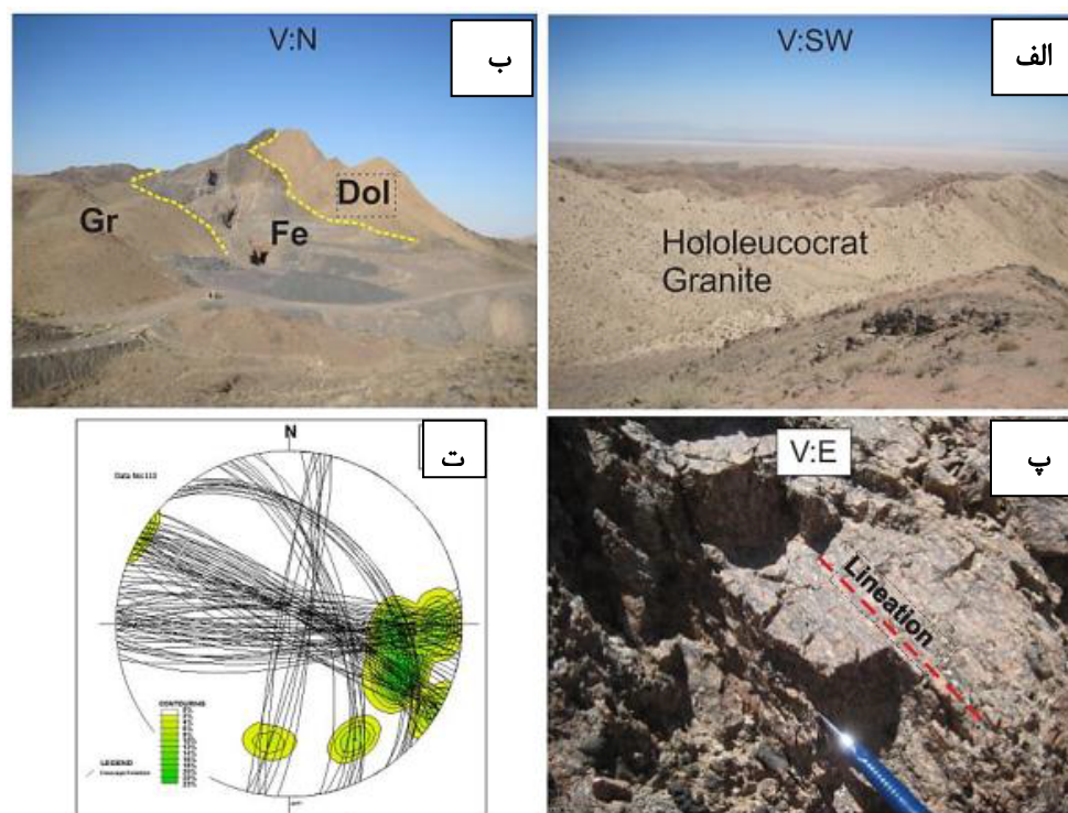
شکل ۴ (الف) گرانیته روشن ده زمان، (ب) سنگ‌شناسی دولومیت و گرانیته در کنار کانسار آهن، (پ) گسترش برگوارگی میلونیته در گرانیته ده زمان، (ت) شکل برجسته‌نگاری برگوارگی در منطقه، (دولومیت: Dol، گرانیته: Gr، آهن: Fe، گرانیته تمام تیره: Hololeucocrat Granite).
