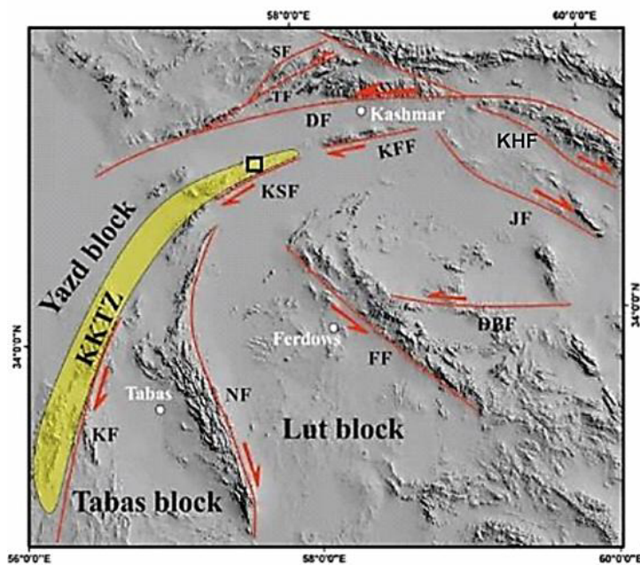
شکل ۱. پهنه‌های ساختاری شرق ایران مرکزی و موقعیت منطقه کوه سرهنگی (مستطیل مشکی‌رنگ): (SF): گسل سبه، (TF): گسل تکرار، (DF): گسل درونه، (JF): گسل تراستی جنگل، (FF): گسل فردوس، (NF): گسل نایبند، (KF): گسل کلمرد، (KHF): گسل خواف، (DBF): گسل دشت بیاض، (KFF): گسل کوه فغان، (KSF): گسل کوه سرهنگی، (KKTZ): پهنه کاشمر- کرمان).
