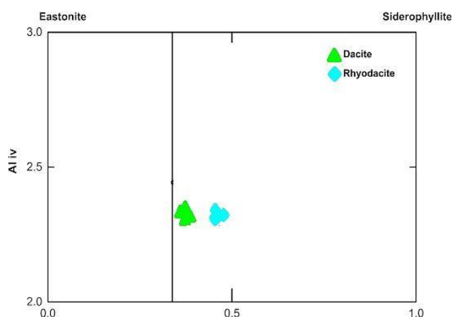
شکل ۷ ترکیب میکاهای نمونه‌های اسیدی منطقه (شامل داسیت و ریوداسیت) در نمودار Fe_t/Fe_t+Mg نسبت به Al_{IV} . که همه آنها با داشتن مقادیر بالای Mg در گستره بیوتیت واقع می‌شوند.
