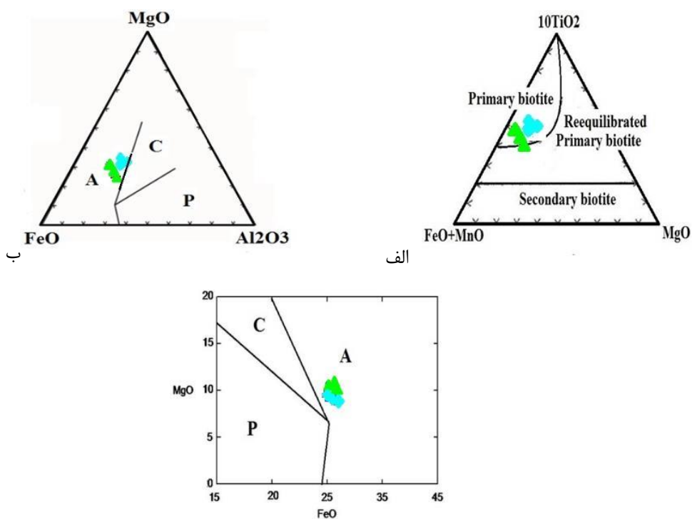
شکل ۸ الف- نمودار تفکیک بیوتیت‌های اولیه، بیوتیت‌های دچار باز تعادل شده و ثانویه [۱۳]. ب و پ- نمودارهای جایگاه زمین‌ساختی گرانیتوئیدها بر اساس ترکیب بیوتیت‌ها [۱] A: الکالین غیرکوهزایی و مناطق کششی، P: سنگ‌های پرآلومین و محیط‌های برخوردی و C: سنگ‌های آهکی قلیایی و مناطق فروورانش.
