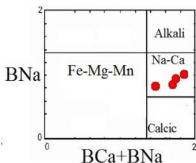
شکل ۶ رده‌بندی آمفیبول‌ها بر پایه ترکیب شیمیایی آنها [۹].
