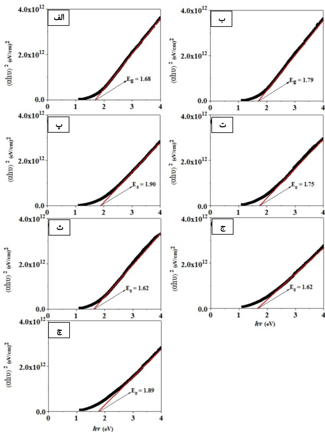
شکل ۹. برون‌یابی قسمت خطی نمودار (\alpha hv)^2 نسبت به (hv) برای نانوذرات Mn_{0/3-x}Ba_xCu_{0/2}Zn_{0/5}Fe_2O_4 با x = 0,00 (الف) تا x = 0,30 (ج). x = 0,05 (پ) x = 0,10 (ت) x = 0,15 (ث) x = 0,20 (ج) x = 0,25 (چ) x = 0,30 .
