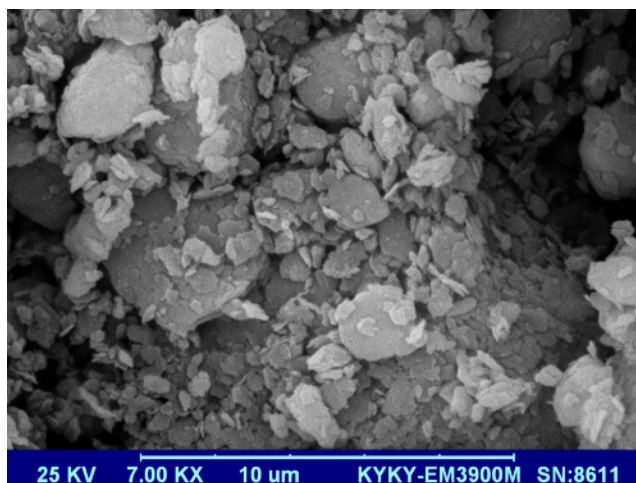
شکل ۷ تصویر میکروسکوپ الکترونی با بزرگنمایی هفت هزار برابر و ولتاژ شتاب دهنده ۲۵ کیلو ولت.
