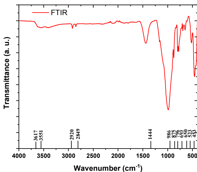
شکل ۱۰ طیف فروسرخ نمونه مورد بررسی.
