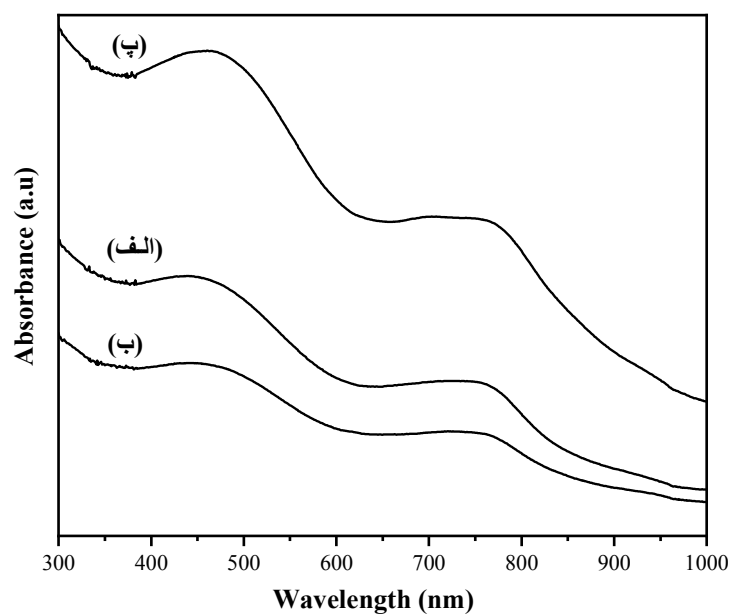
شکل ۴: طیف‌های جذبی UV-Vis نانو ذرات اکسید کبالت تهیه شده با مایع یونی در غلظت‌های متفاوت NaOH (الف) ۱ میلی مول، (ب) ۲ میلی مول و (پ) ۳ میلی مول.
