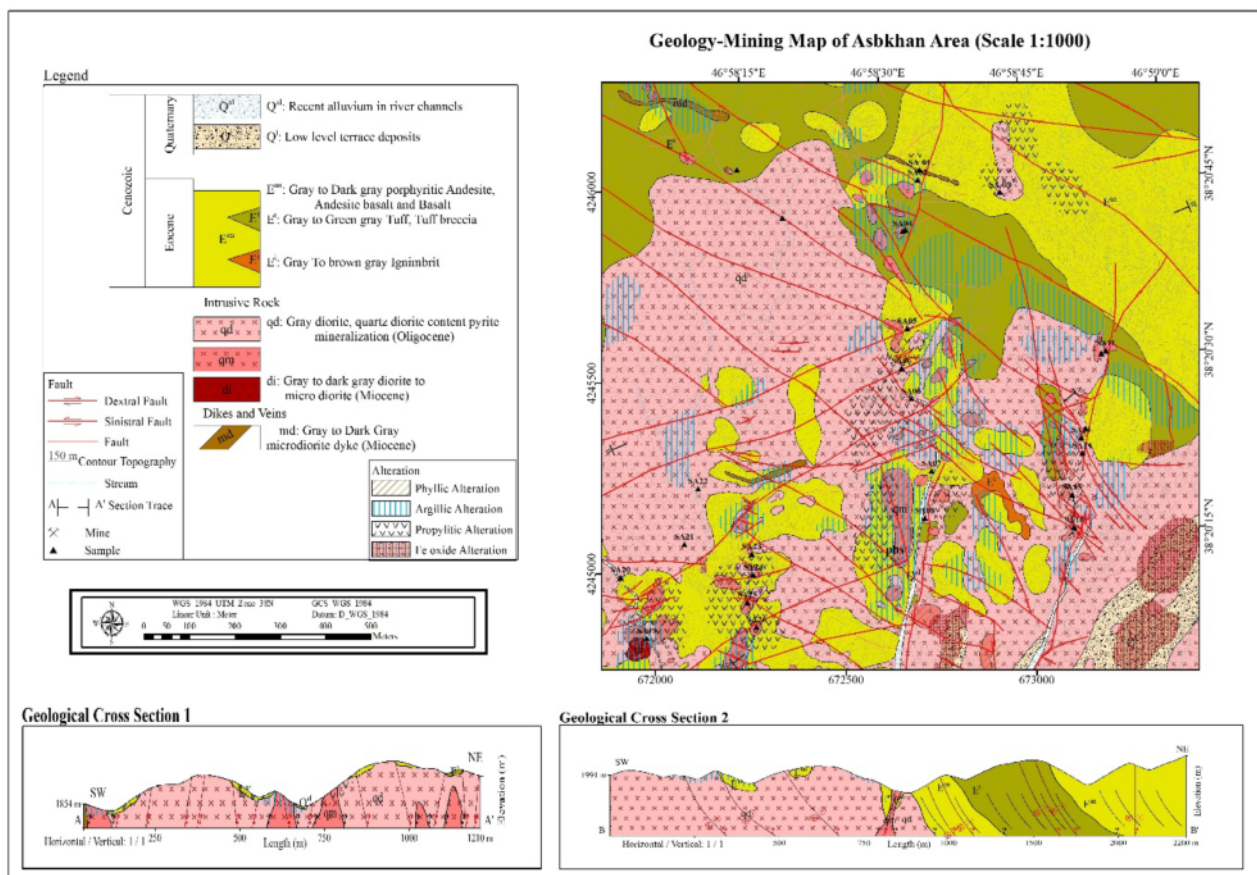
شکل ۲ نقشه زمین شناسی منطقه اسبخان در مقیاس ۱:۱۰۰۰ برگرفته از مراجع [۲۶، ۲۵] با تغییرات.
