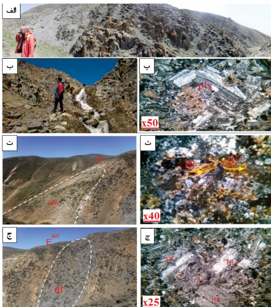
شکل ۳ الف) نمای دور از واحد کوارتز-دیوریتی با دید به سمت شرق، ب) نمای نزدیک از واحد کوارتز-دیوریتی، پ) مجموعه‌ای از درشت بلورهای دانه درشت تا متوسط پلاژیوکلاز و ارتوز (در نور قطبیده متقاطع XPL)، ت) نمایی از مرز واحد کوارتز-مونزونیت پورفیری با توده کوارتز-دیوریت، ث) تصویری از تشکیل بیوتیت ثانویه در توده کوارتز-مونزونیت پورفیری (در نور XPL)، ج) نمایی از توده دیوریتی تا میکرودیوریتی که به شکل دایک در توالی ائوسن نفوذ کرده است، چ) تصویری از بافت دانه‌ای به همراه پلاژیوکلاز و فلدسپار قلیایی موجود در توده دیوریتی (در نور XPL).
