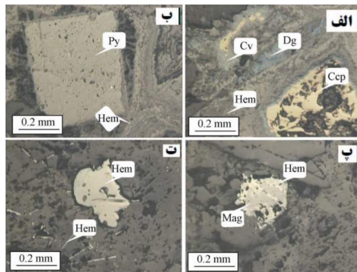
شکل ۶ تصاویر میکروسکوپی (در نور بازتابی) از کانی‌های فلزی ذخیره لپه‌زنک: الف) جانشینی کالکوپیریت توسط کانی‌های ثانویه دیژنیت، کوولیت و هماتیت، ب) جانشینی کامل پیریت توسط هماتیت که تنها قالبی از پیریت باقیمانده است، پ) اورالیتی شدن مگنتیت و تبدیل بخشی آن به هماتیت، ت) رخدادهای کانی‌های ورقه‌ای و سوزنی‌شکل هماتیت در کانسنگ. Py: پیریت، Ccp: کالکوپیریت، Cv: کوولیت، Dg: دیژنیت، Mag: مگنتیت و Hem: هماتیت [۱۰].
