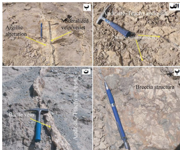
شکل ۴ (نمایی از الف) رگه-رگچه‌های کوارتزی در واحد آندزیت- تراکی آندزیت، (ب) دگرسانی آرژیلیک رسی پیرامون رگه-رگچه‌های شامل کانه‌زایی. (پ) ساختار برشی در رگه باریتی و (ت) رخنمونی از رگه باریتی در واحد آندزیت- تراکی آندزیت در منطقه لپه‌زنک.
