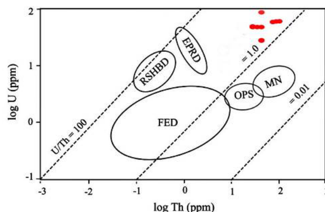
شکل ۸ نمودار تفکیک کننده U نسبت به Th [۱۵]. FED: ذخایر برون‌دیمی سنگواره، OPS: رسوب‌های گودابه‌ای متداول، MN: گرهک‌های منگنز، RSHBD: ذخایر آبشور دریای سرخ و EPRD: ذخایر پشته‌های میان اقیانوس آرام.
