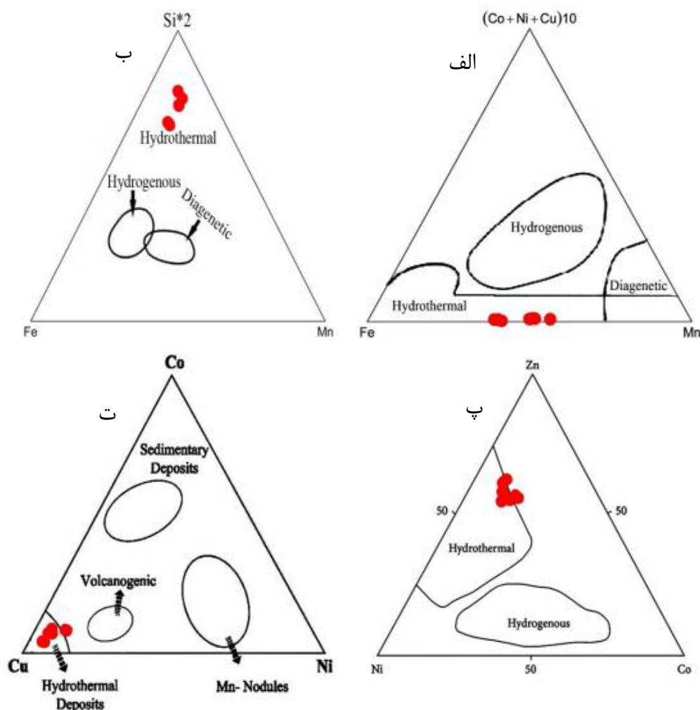
شکل ۶ نمودارهای سه‌تایی الف) 10 \times (\text{Fe} + \text{Mn} + (\text{Co} + \text{Ni} + \text{Zn})) [۶]، ب) \text{Fe} - \text{Mn} - \text{Si} \times 2 [۳۱]، پ) \text{Zn} - \text{Co} - \text{Ni} [۳۳] و ت) \text{Cu} - \text{Co} - \text{Ni} [۳۴] و قرارگیری نمونه‌های منطقه مورد بررسی در بخش گرمابی.
