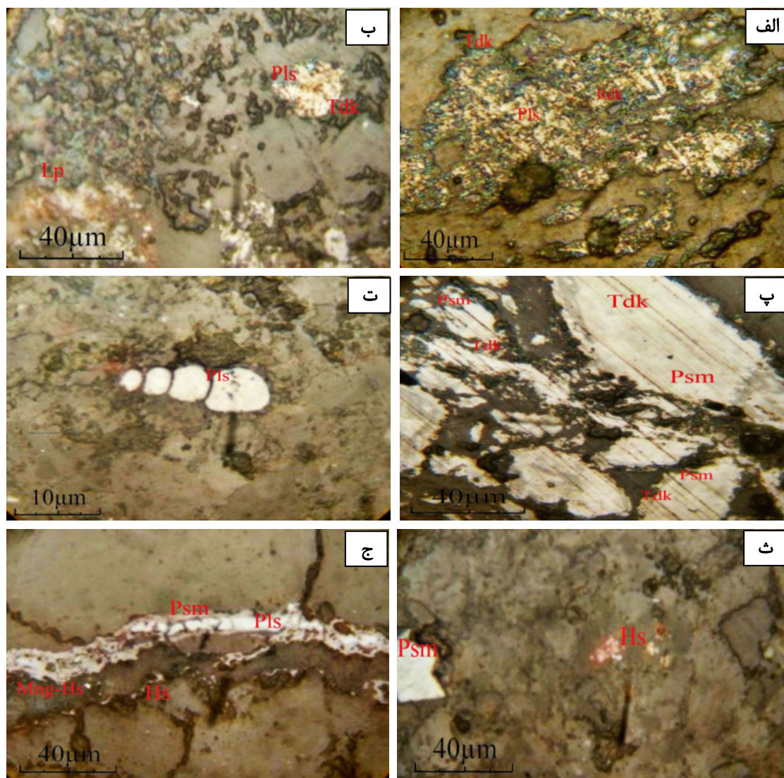
شکل ۴ الف)-نمایی از پیرولوسیت (Pls) در حال دگرسانی به تودوروکیت (Tdk). ب) کانی پیرولوسیت (Pls) در حال دگرسانی به تودوروکیت (Tdk) و لپیدوکروزیت (Lp). پ) پسیلوملان‌های (Psm) کمی دگرسان شده به تودوروکیت (Tdk). ت) جانشینی پیرولوسیت (Pls) دگرسان شده در قالب ریز سنگواره. ث) هوسمانیت (Hs) ریزبلور در کنار بلور پسیلوملان. ج) نمایی از سیلیس، کربنات و اکسید-هیدروکسیدهای منگنز-پیرولوسیت (Pls) دگرسان شده به پسیلوملان (Psm)، هیدروهوسمانیت (Ho)، مانگانیت (Mng).
