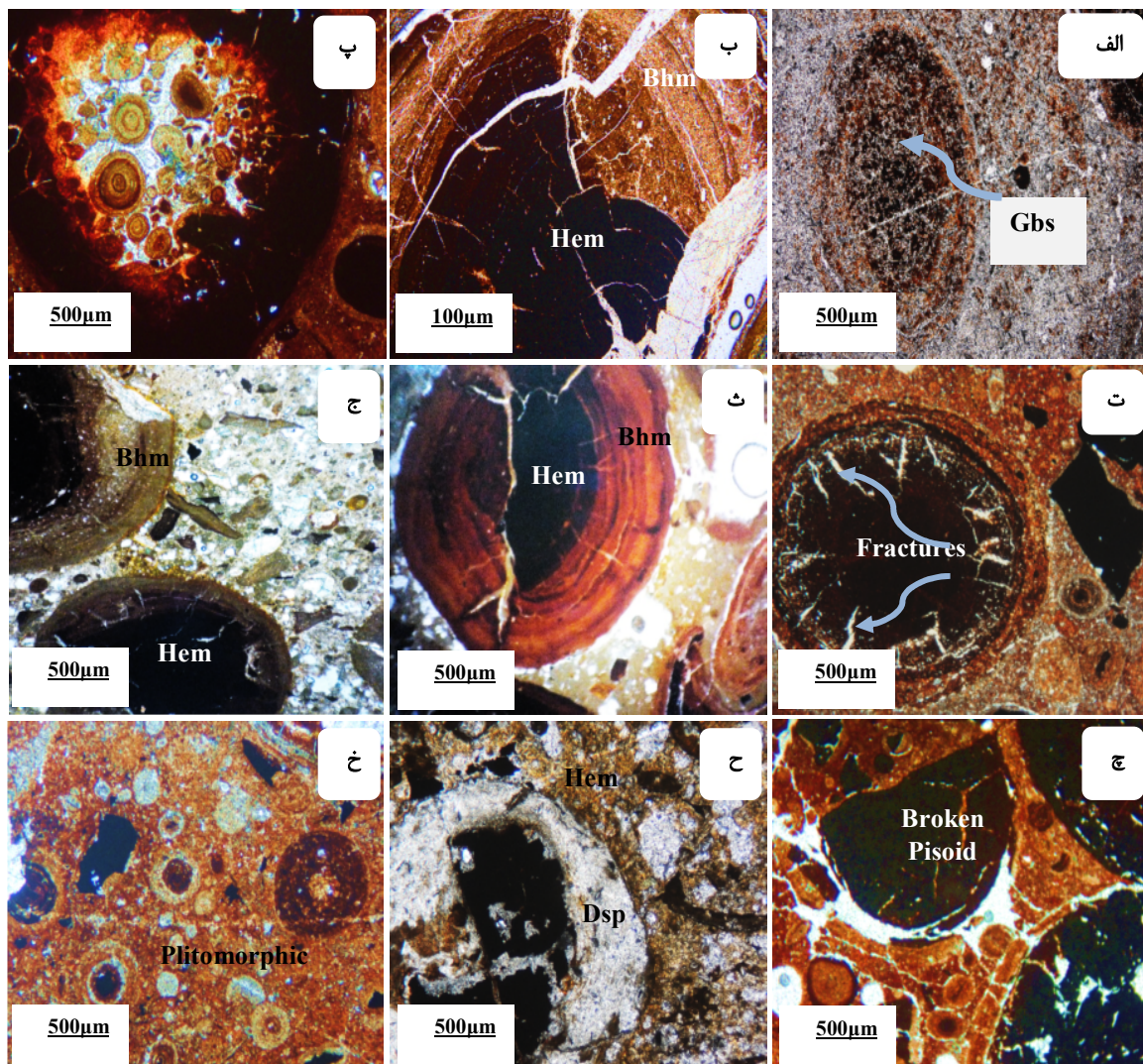
شکل ۶ تصاویر میکروسکوپی نهشته بوکسیتی پیراشکفت: (الف) کانی گیبسیت در بافت تخریبی شدید (4x)، (ب) پیزوئید با ترک های انقباضی (10x)، (پ) هسته اووئیدی در پیزوئید بزرگ (4x)، (ت) شکستگی های شعاعی ناشی از تزریق ژل در پیزوئیدهای نیمه خرد شده (4x)، (ث) پیزوئید تشکیل شده با لایه هایی از اکسید آهن و اکسید آلومینیوم پس از شکستگی پیزوئید بر اثر تزریق ژل، (ج) پیزوئید برجوازاد (4x)، (چ) پیزوئید دگرزاد داخل ماتریکس میکروگرانولار (4x)، (ح) هسته آواری شکسته که پیرامون آن لایه هایی از دیاسپور تشکیل شده است (4x) و (خ) بافت اووئیدی (4x). همه تصاویر در نور قطبیده متقاطع، xpl، ثبت شده اند. (هماتیت = Hem، بوهمیت = Bhm، دیاسپور = Dsp، گیبسیت = Gbs).
