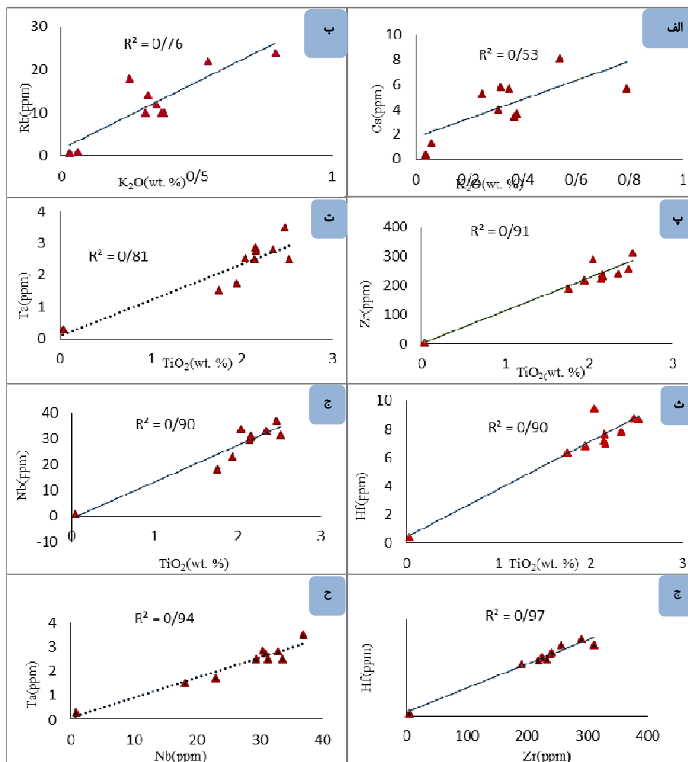
شکل ۱۰ نمودارهای دوتایی ضرایب همبستگی: الف) نمودار Cs نسبت به K_2O (ب) نمودار Rb نسبت به K_2O (پ) نمودار Ti نسبت به Zr (ت) نمودار Ta نسبت به TiO 2 (ث) نمودار Hf نسبت به TiO 2 (ج) نمودار Nb نسبت به TiO 2 (چ) نمودار Zr نسبت به Hf (و) نمودار Nb نسبت به Ta.
