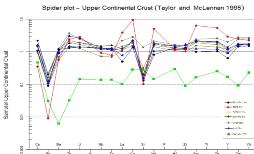
شکل ۱۱ الگوی توزیع عناصر جزئی نمونه‌های بوکسیتی پیراشکفت نسبت به پوسته قاره‌ای بالایی [۱۸].
