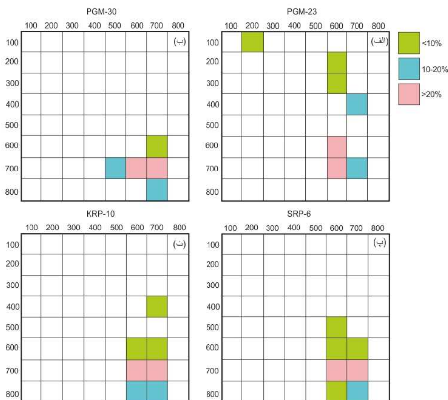
شکل ۹ فراوانی بلورهای زیرکن نمونه‌های اسیدی جنوب شرق سقز بر روی نمودار ریخت‌شناسی مرجع [۱].
