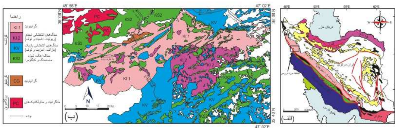
شکل ۱ الف) نقشه ساده شده پهنه‌های زمین‌شناسی ایران [۱۸]، ب) نقشه تصحیح شده منطقه مورد بررسی برگرفته از مراجع [۲۰-۲۵].
