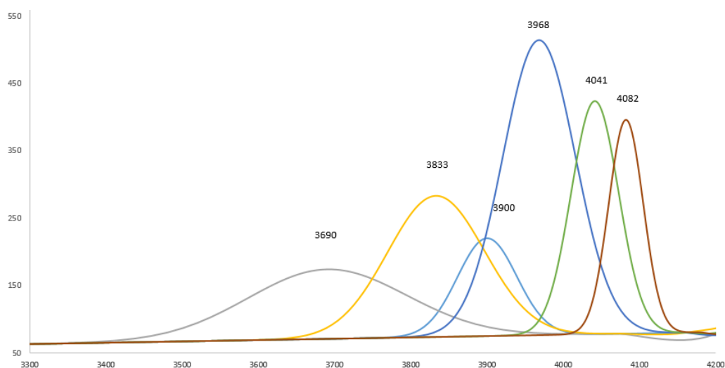
شکل ۳ طیف رامان بیوتیت ششگوشی بروجرد در گستره ۳۳۰۰ تا ۴۲۰۰ cm -1 .
