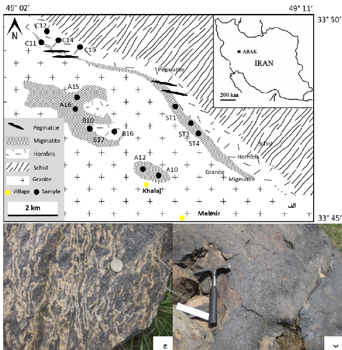
شکل ۱ الف) موقعیت جغرافیایی منطقه مورد بررسی اراک، ایران، ۲۵ کیلومتری بروجرد در منطقه بین غره‌داش و غره‌تپه، ب) رخنمون هورنفلس و پ) رخنمون میگماتیت‌ها.
