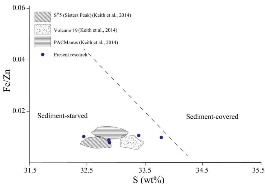
شکل ۷ نمودار درصد وزنی گوگرد نسبت به Fe/Zn در اسفالریت [۲۰]. که براساس آن، اسفالریت‌های موجود در کانسار چشمه نقره شبیه اسفالریت‌های تشکیل‌شده در کانسارهای درون حوضه کم رسوب هستند. بر این اساس، دمای تشکیل اسفالریت‌های کانسار چشمه نقره حدود ۲۳۵ درجه سانتیگراد است.
