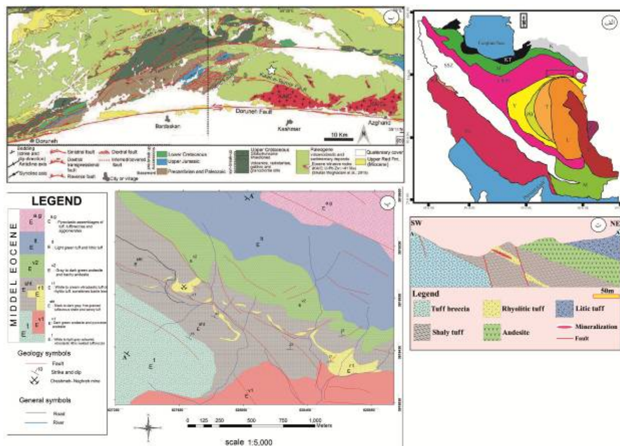
شکل ۱ الف) نقشه زمین‌شناسی ساختاری ایران [۱۹،۱۸]. ب) نقشه زمین‌شناسی زیرپهنه سبزوار. پ) نقشه زمین‌شناسی کانسار چشمه نقره. ت) مقطع عرضی کانسار چشمه نقره که موقعیت آن با علامت ستاره نقشه زمین‌شناسی تصاویر الف و ب نشان داده شده است.
